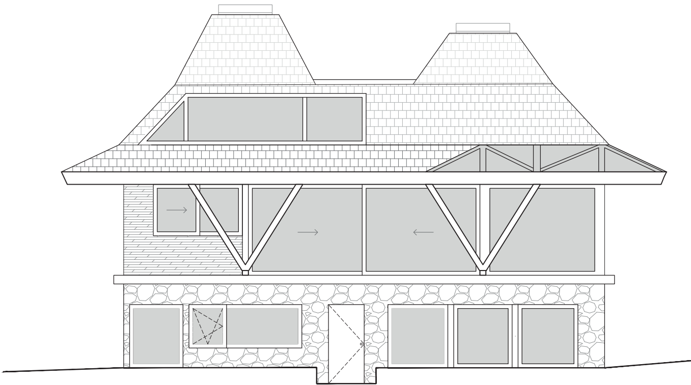
ELEVACIÓN SUR
