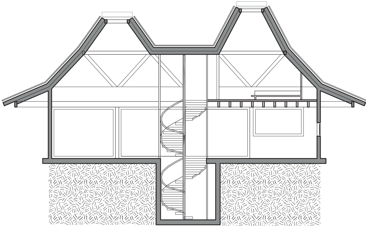
CORTE LONGITUDINAL
