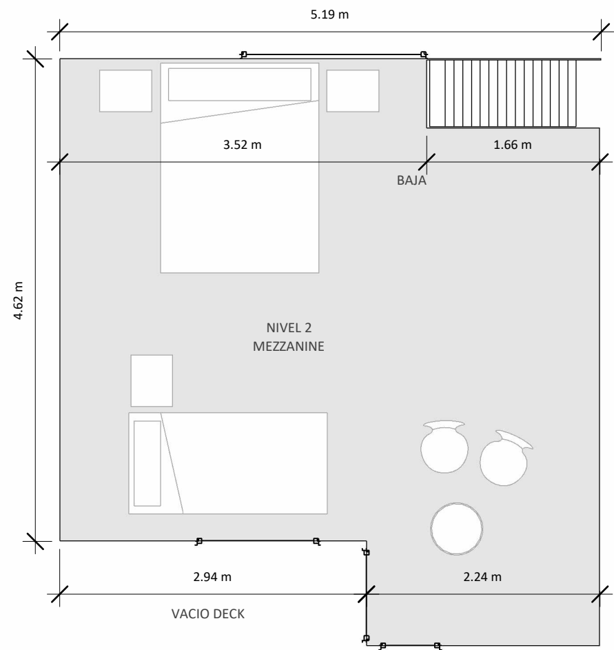
2 Nivel 2 1 : 50
