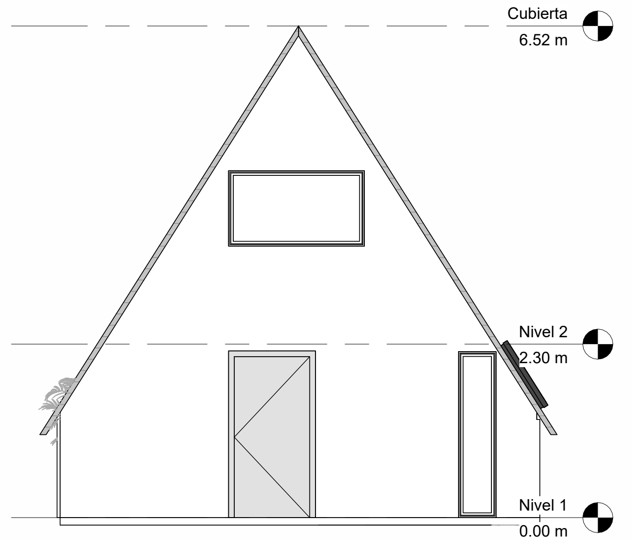
5 Fachada Norte 1 : 50
