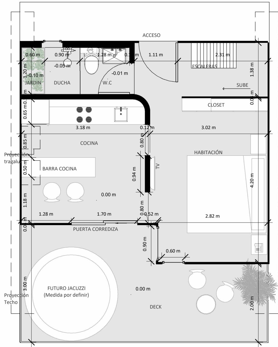
1 Nivel 1 1 : 50
