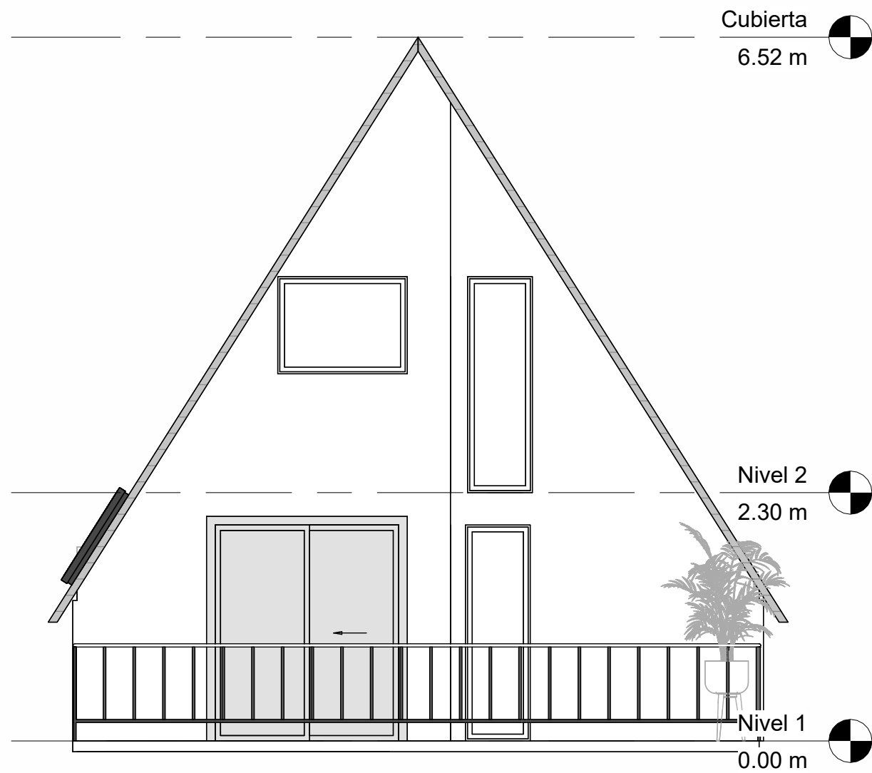
3 Fachada Sur 1 : 50
