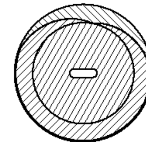
DETALLE A-A ESCALA 2 : 1
