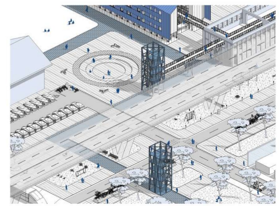
Isométrica detalle 4 / Torres y anfiteatro público esc. 1:400
