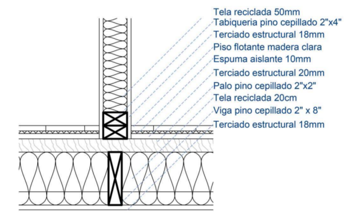
Detalle constructivo B / esc. 1:10
