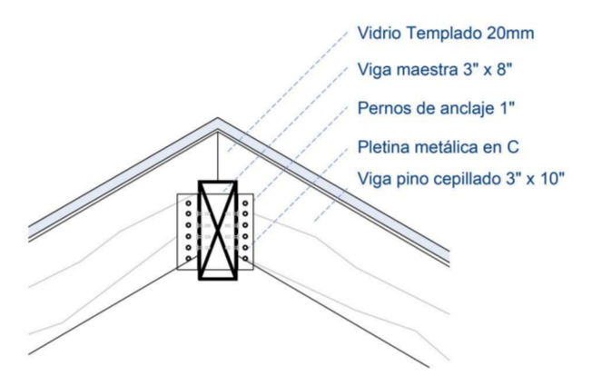
Detalle constructivo A / esc. 1:10
