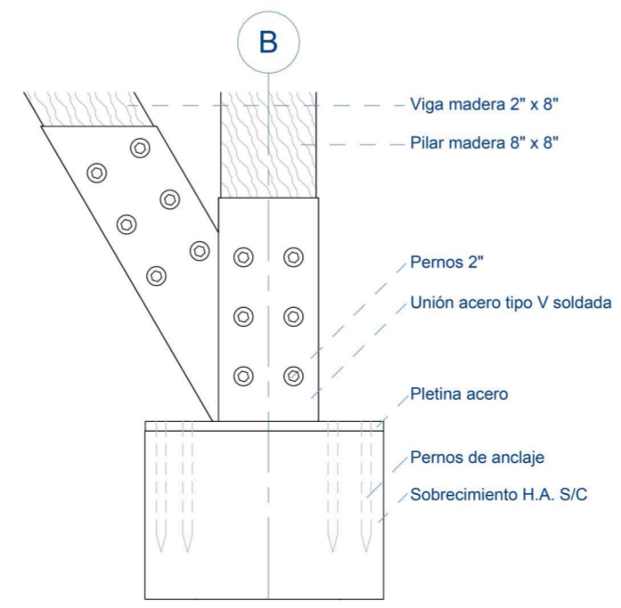
Detalle constructivo C / esc. 1:10
