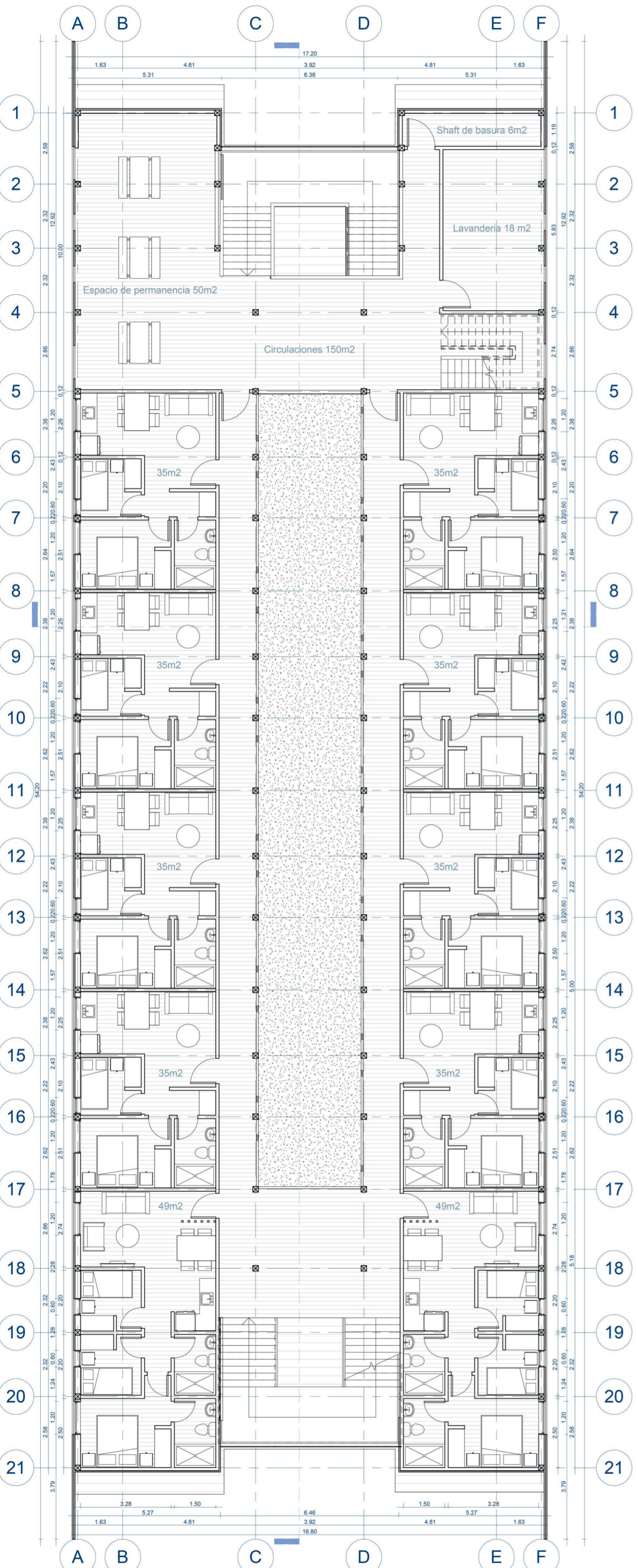
Planta tipo nivel 2 / esc. 1:100
