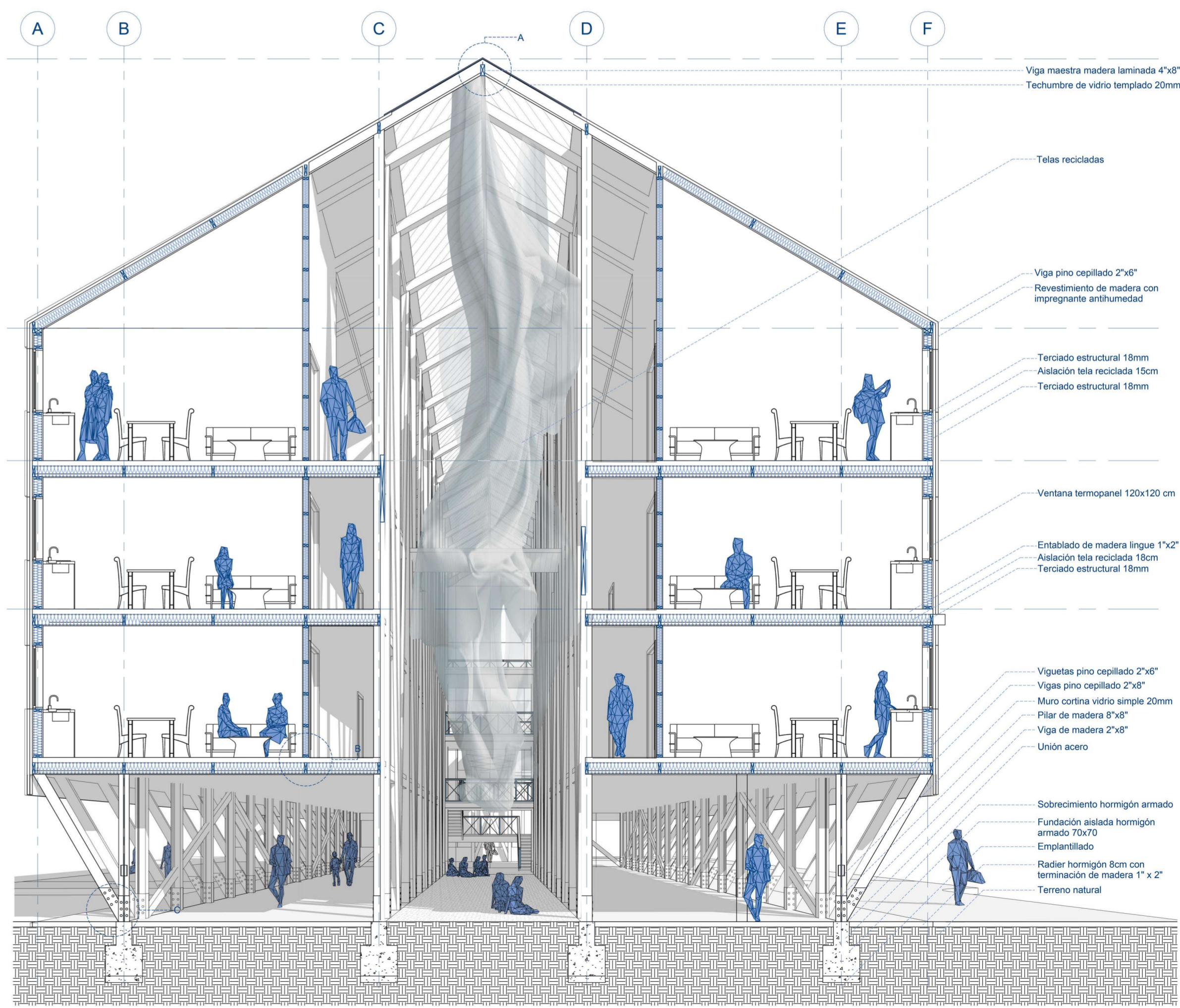
Corte constructivo / esc. 1:50
