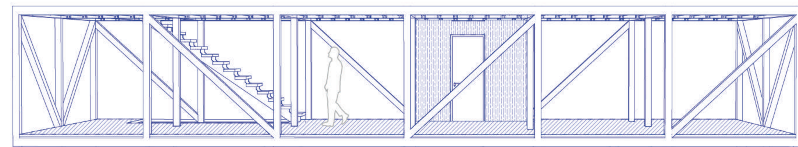
ELEVACIÓN EN PERSPECTIVA DEL SEGUNDO PISO
