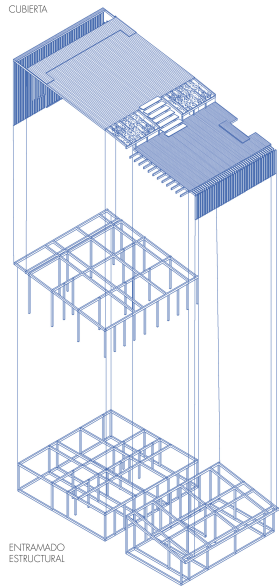
ISOMETRICA EXPLOTADA ESTRUCTURA ESC. 1/100
