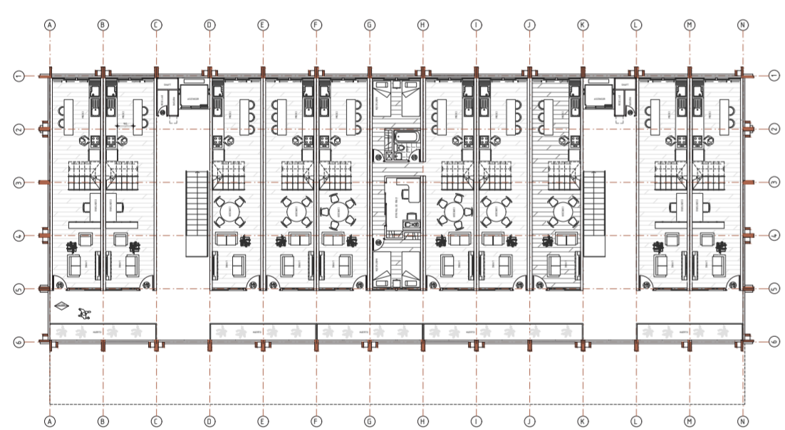
PLANTA ARQUITECTURA NIVEL 2 Y 4 - PABELLÓN TIPO
