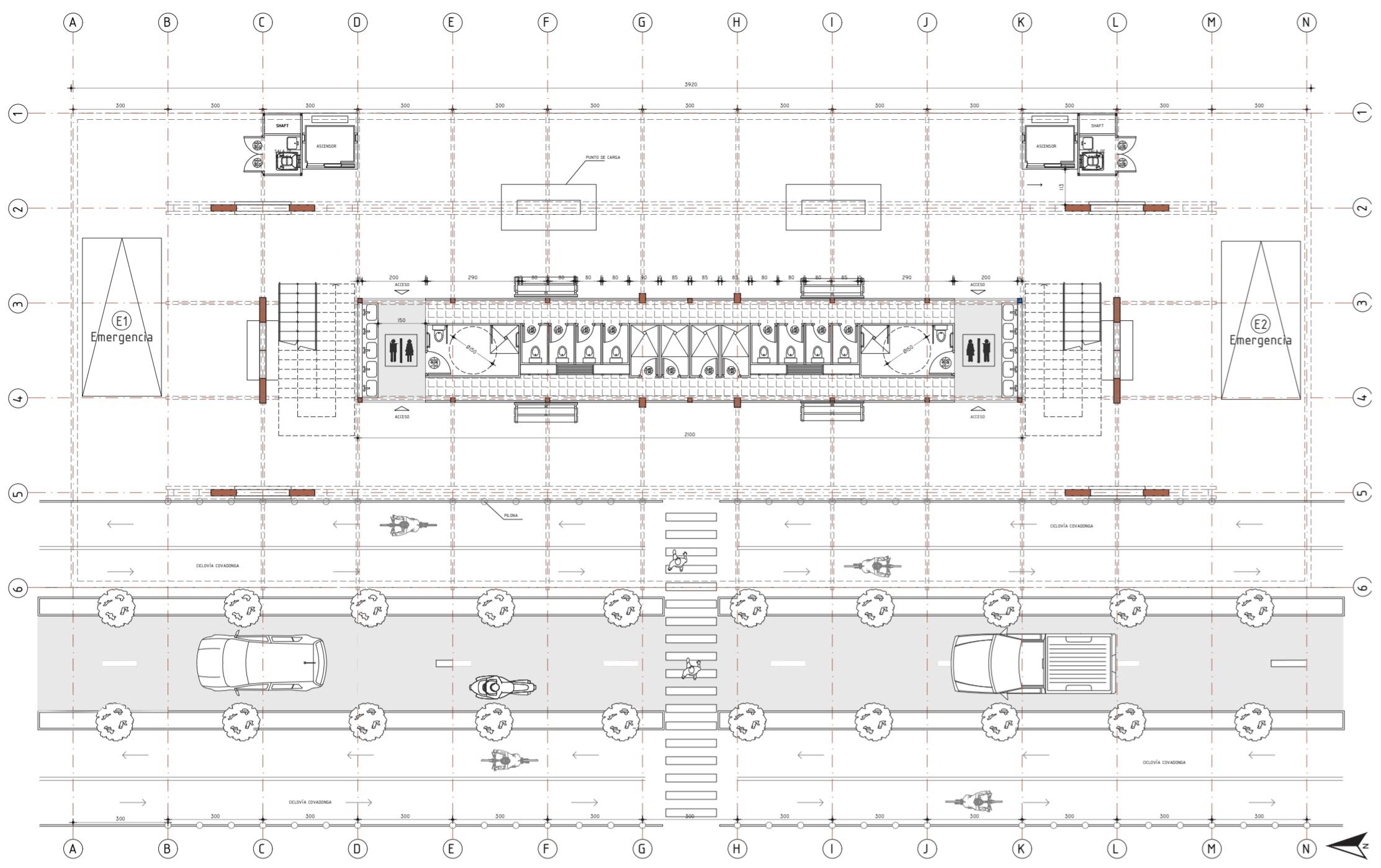
PLANTA ARQUITECTURA NIVEL 1 - PABELLÓN TIPO
