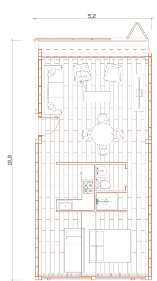
PLANTA DEPARTAMENTO PEQUEÑO 42 m 2 ESC 1:50
