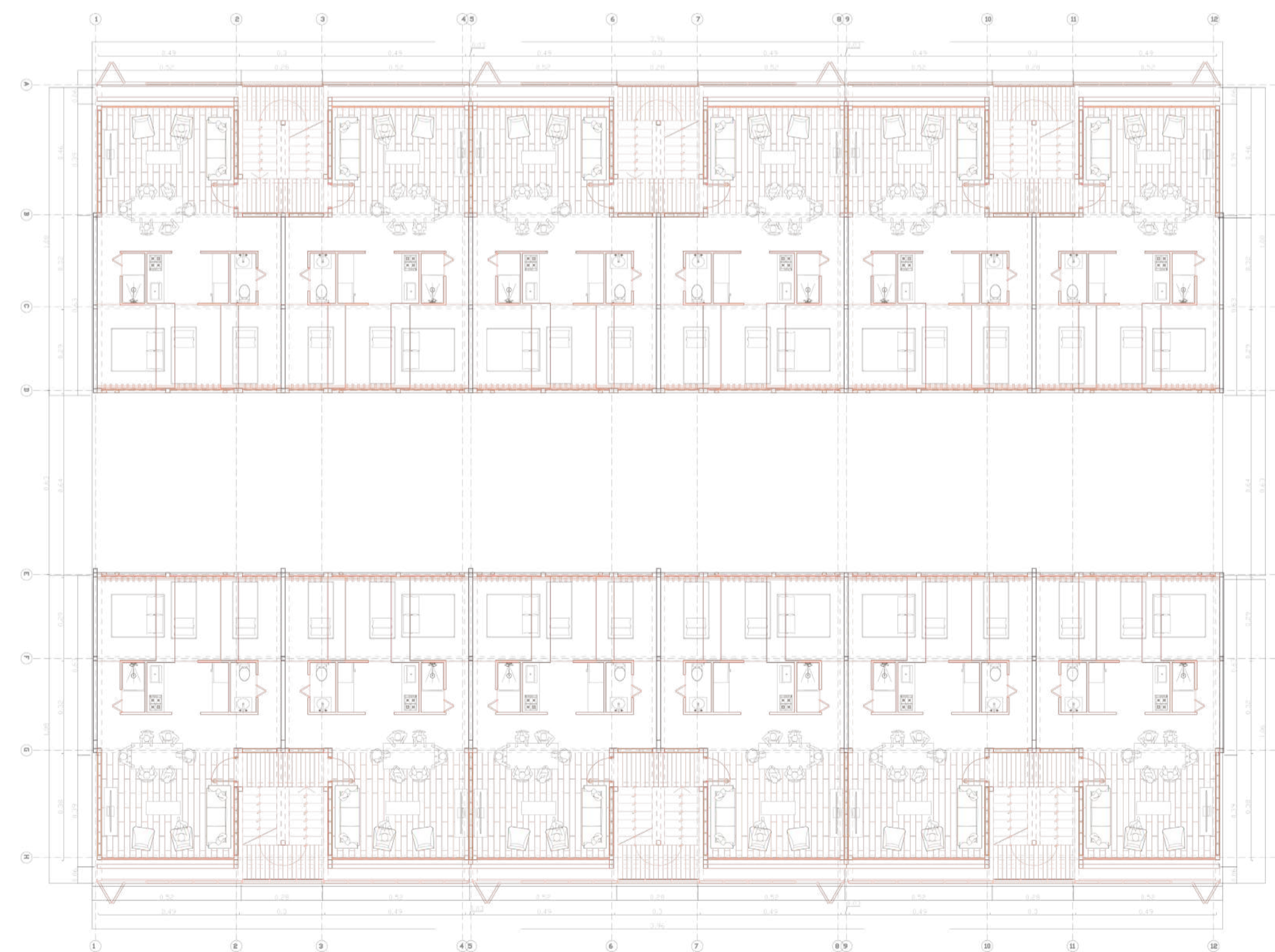
PLANTA PRIMER PISO (NIVEL CALLE) ESC 1: 100
