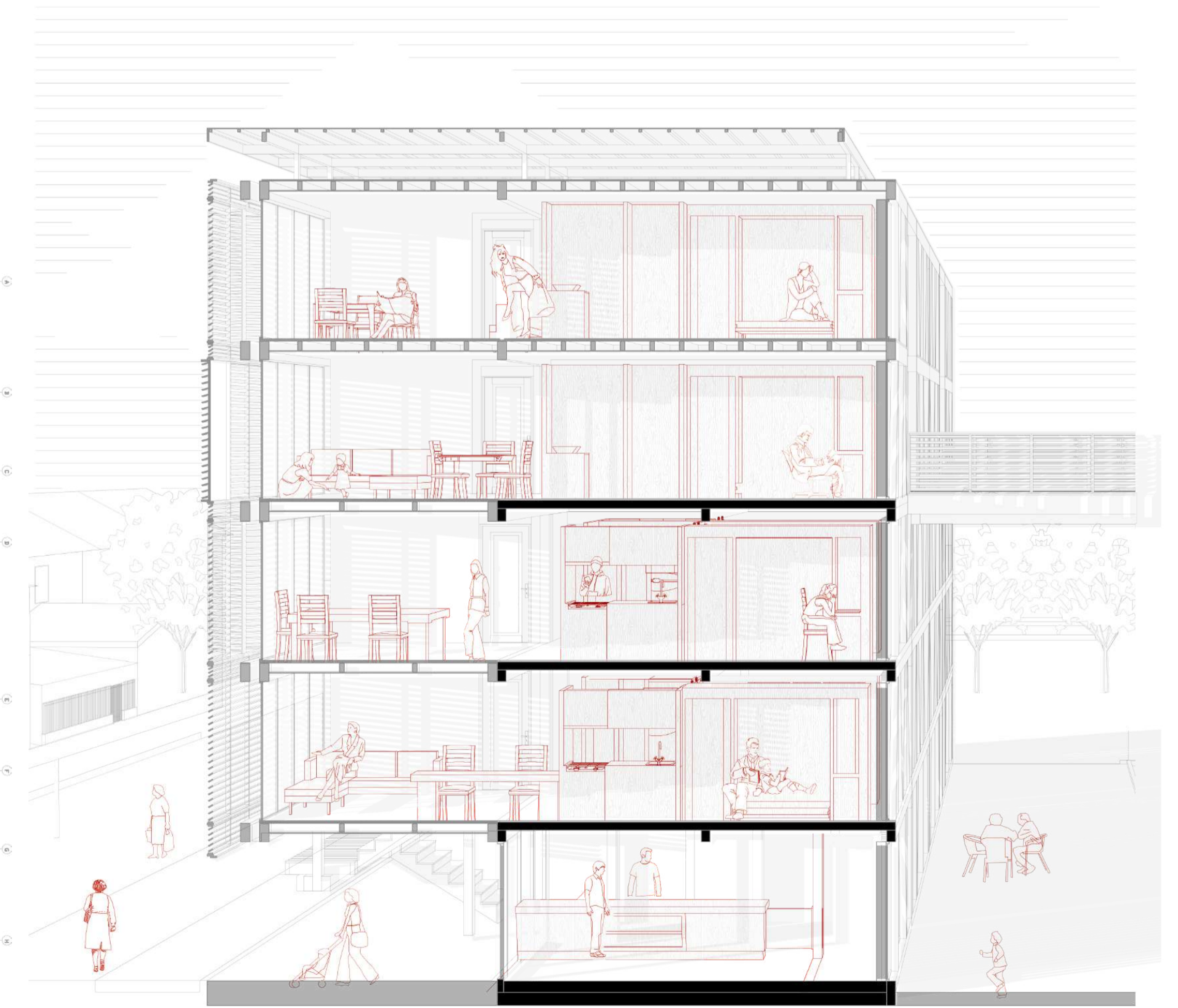
CORTE DE BLOCK QUE MIRA A LA CALLE. ESC 1:50
