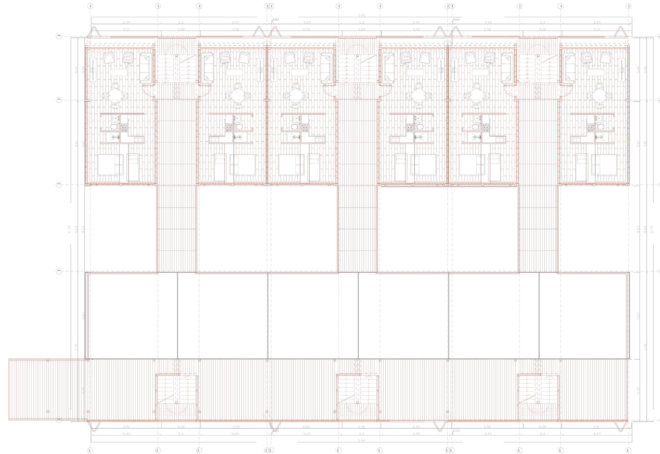
PLANTA TERCER PISO (NIVEL TERRAZA) ESC 1: 100
