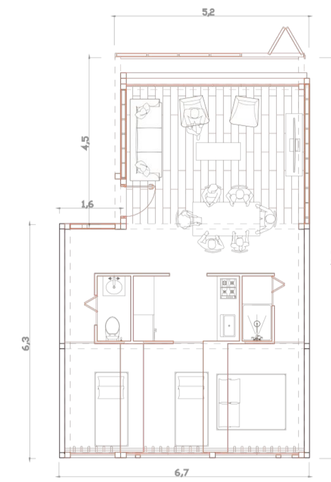
PLANTA DEPARTAMENTO GRANDE 66 m 2 ESC 1:50
