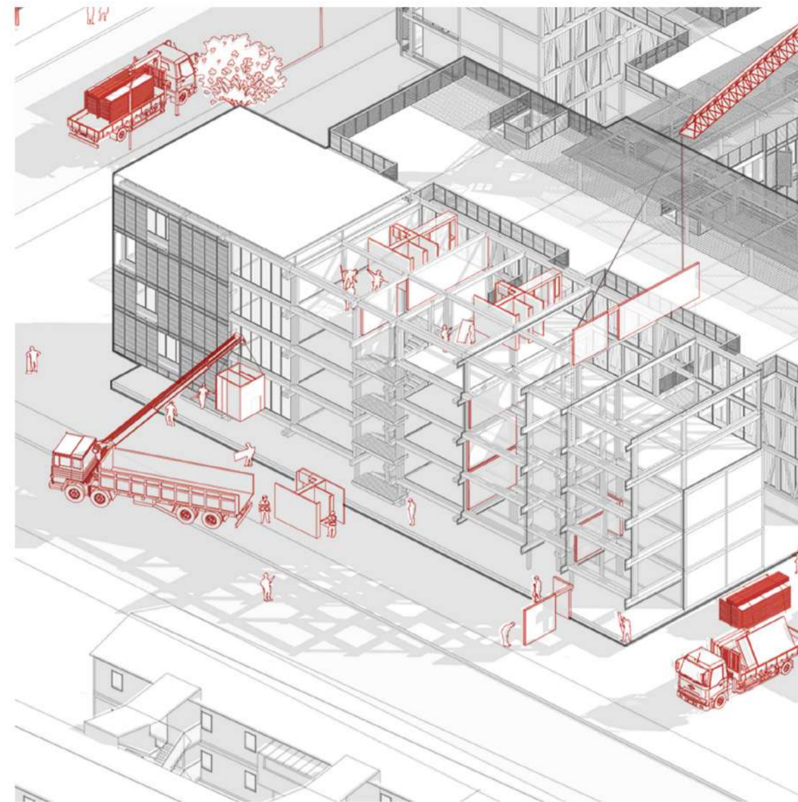
2.- Proceso constructivo. Por medio de una estructura modular se amplian los departamentos pre-existentes, encajando cerramientos perimetrales de paneles de madera laminada pre-fabricada CLT; estos contendrán una nueva distribución residencial, donde los recintos estarán concentrados en un "mueble".
