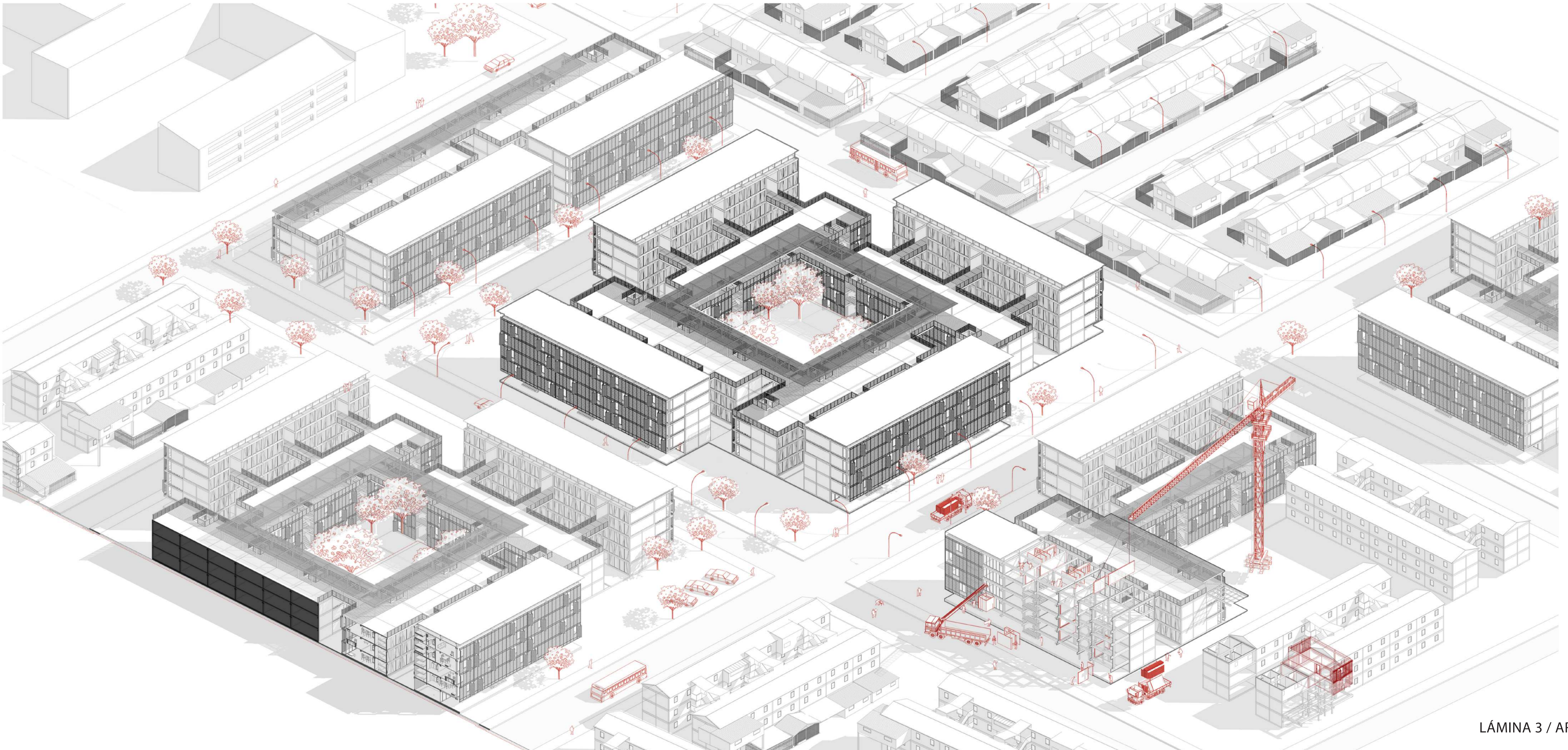
2.- Proceso constructivo. Por medio de una estructura modular se amplian los departamentos pre-existentes, encajando cerramientos perimetrales de paneles de madera laminada pre-fabricada CLT; estos contendrán una nueva distribución residencial, donde los recintos estarán concentrados en un "mueble".
