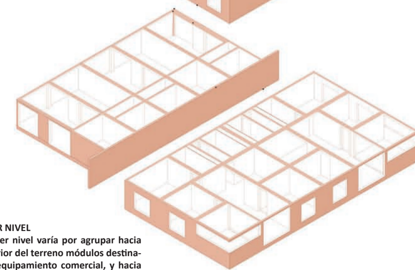
VIVIENDAS Las viviendas se agrupan alrededor del bloque central de circulación.
