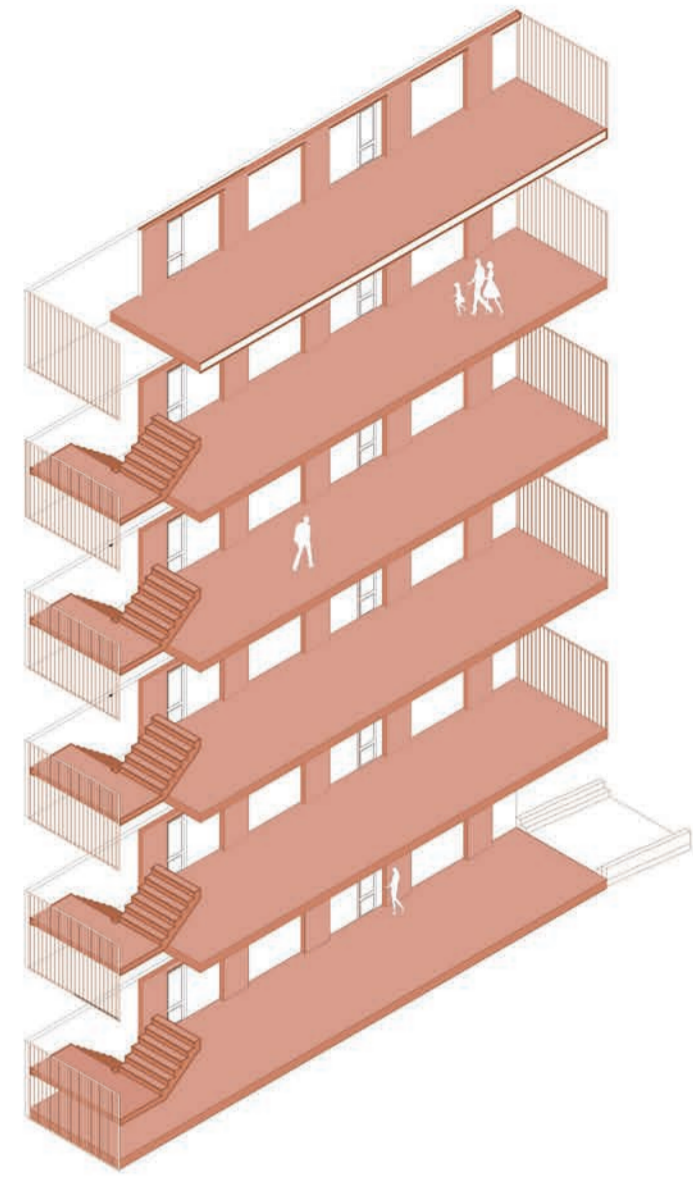
Piezas de los módulos de circulación
