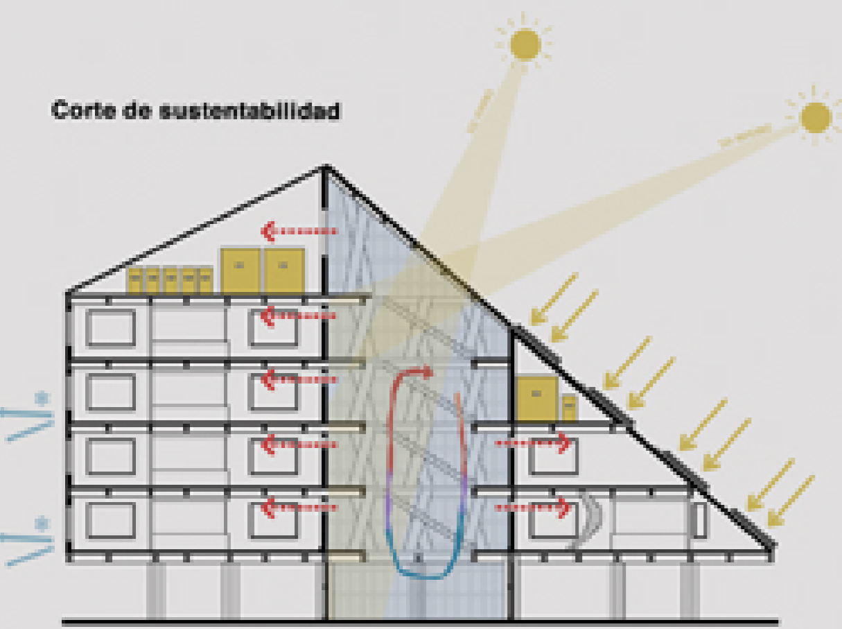
Corte A-A' 1:300
