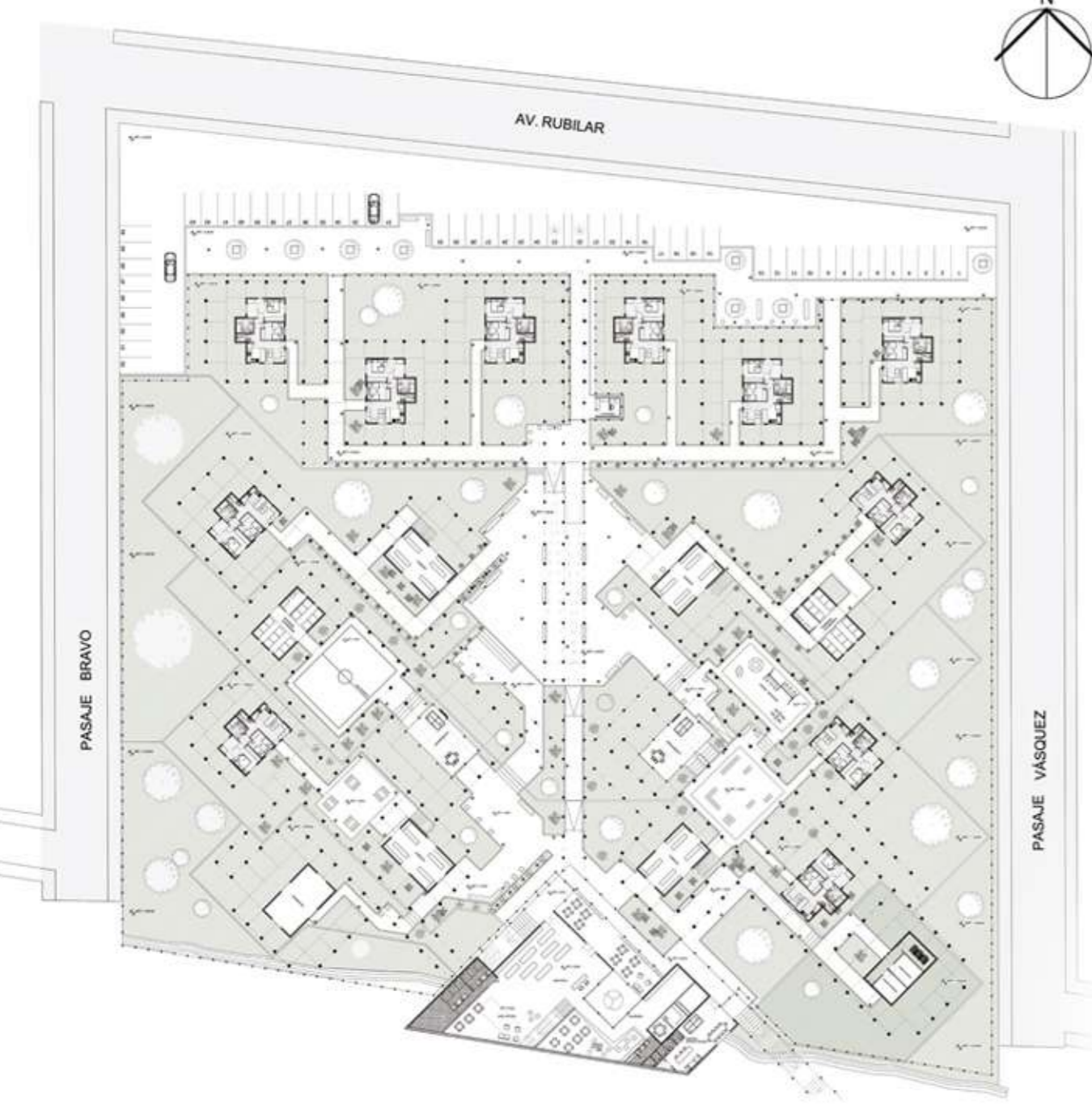
Planta Primer Nivel Espacio Publico - Equipamiento barrial
