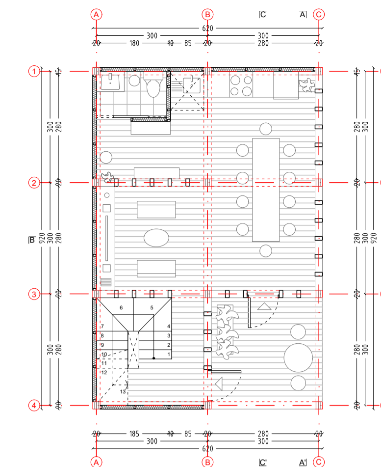
PLANTA PRIMER NIVEL | 1:100
