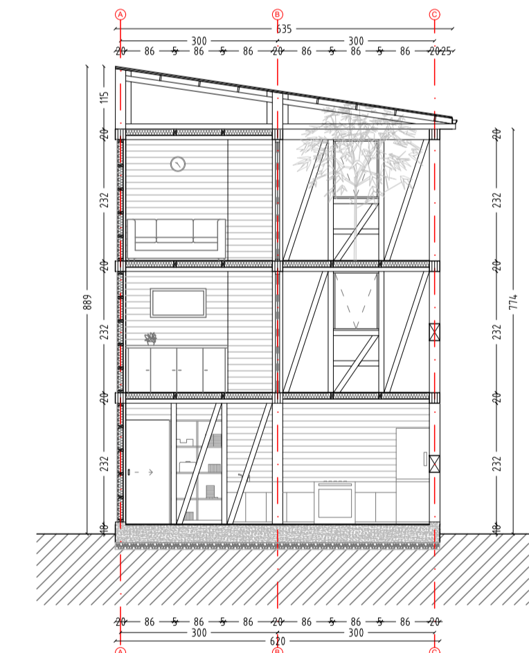
CORTE B-B' | 1:100
