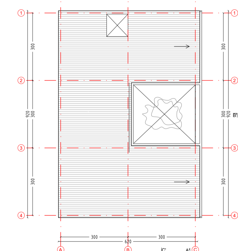
PLANTA CUBIERTA | 1:100
