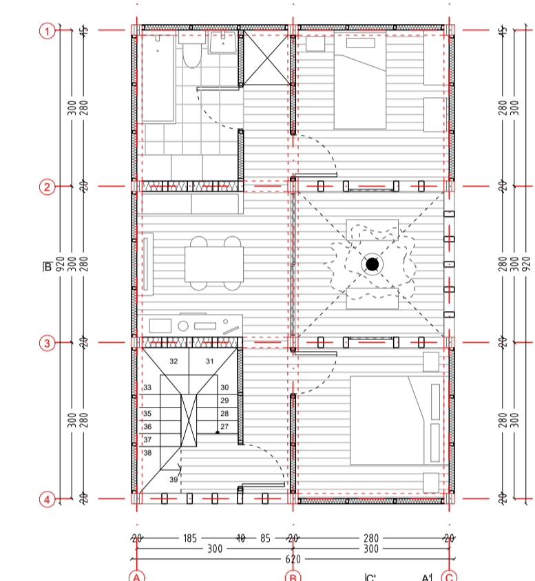
PLANTA TERCERO NIVEL | 1:100
