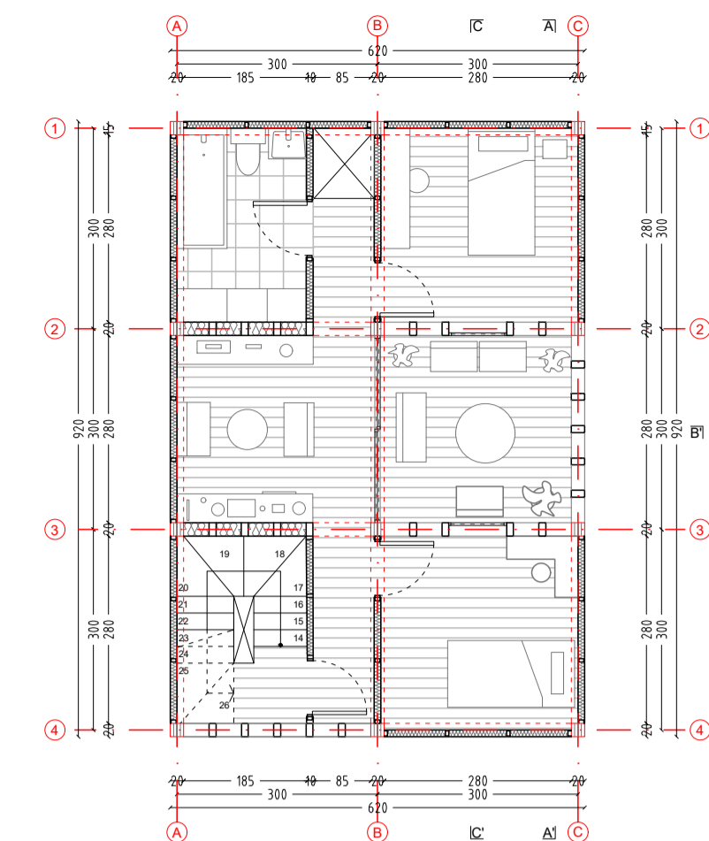
PLANTA SEGUNDO NIVEL | 1:100
