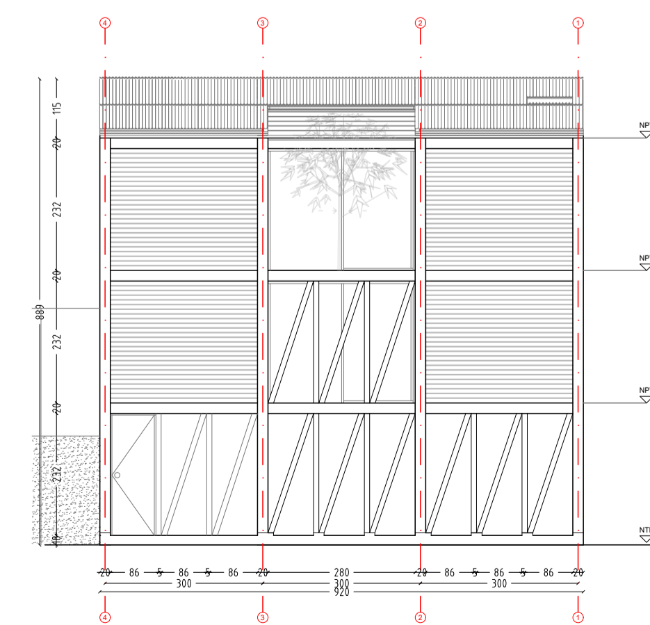
ELEVACION FRONTAL | 1:100
