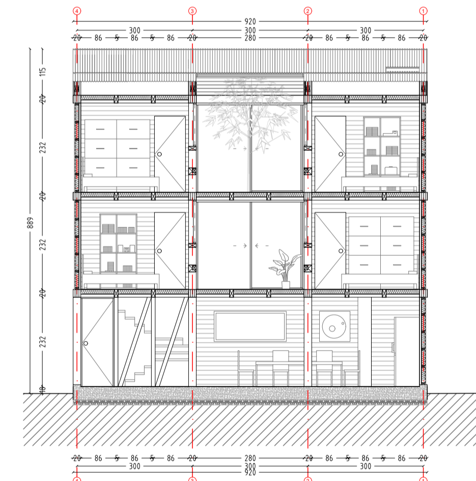
CORTE A-A' | 1:100
