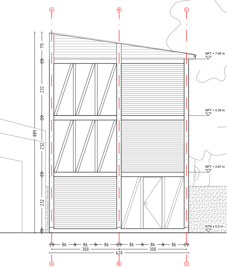
ELEVACION LATERAL | 1:100
