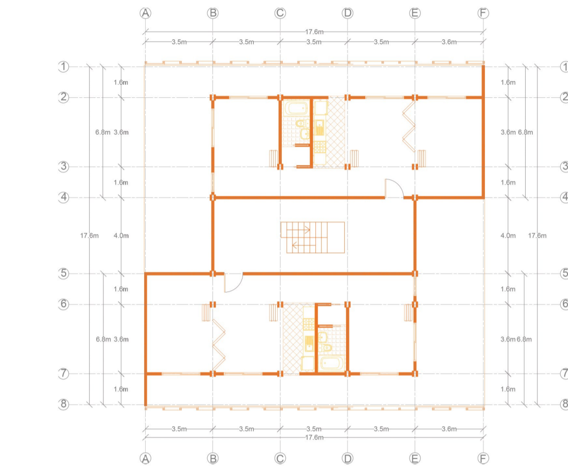
Planimetría barrial intermedia 2.
