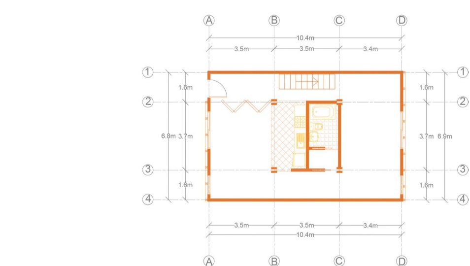
Planimetría barrial duplex 4.
