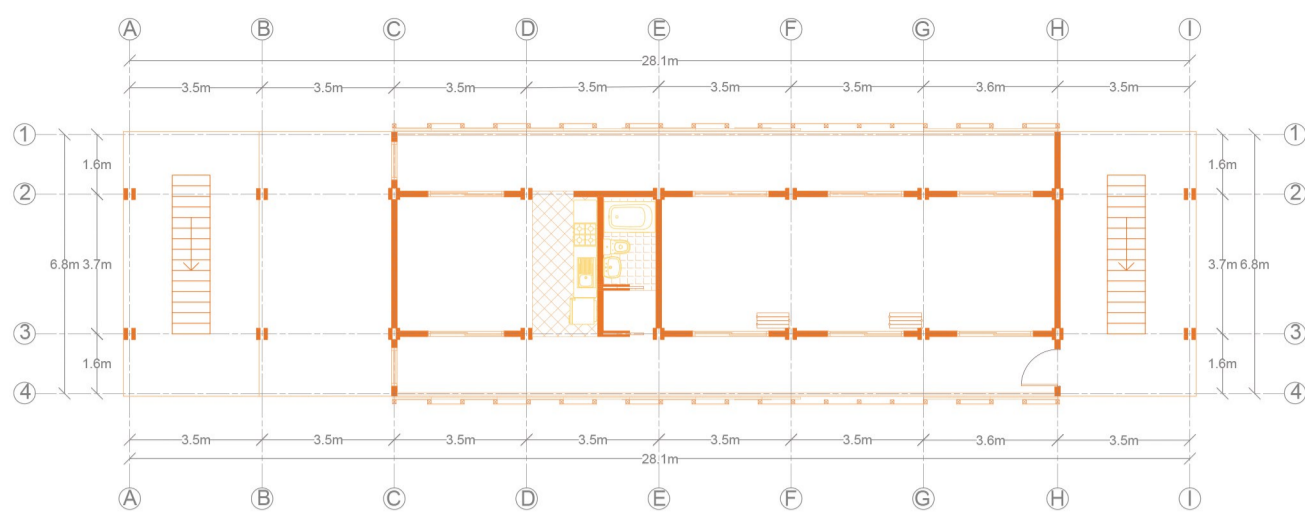
Planimetría metropolitana 1
