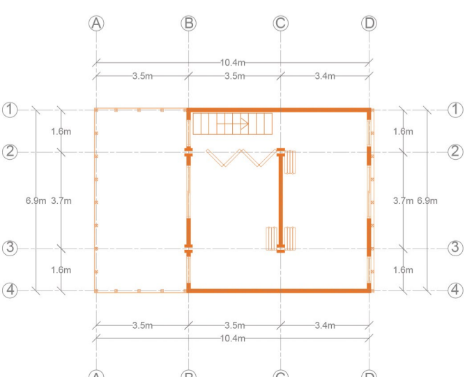
Planimetría barrial duplex 4.
