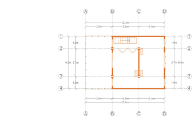
Planimetría barrial duplex 4. Escala 1:200.
