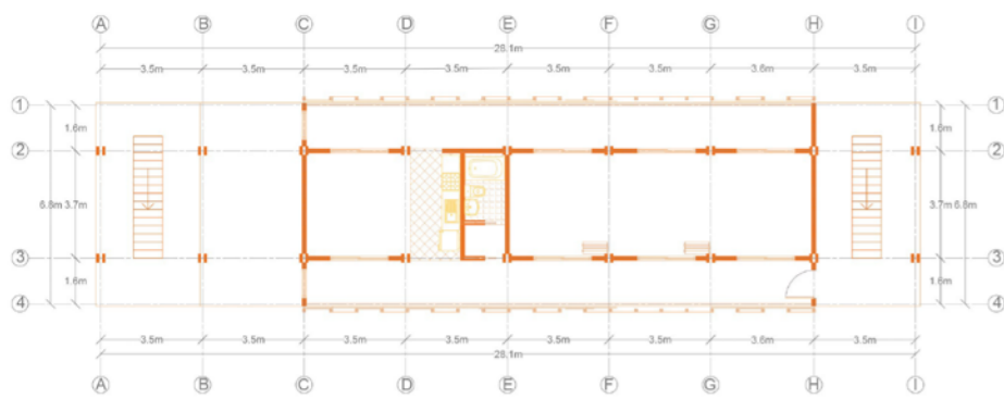
Planimetría metropolitana 1 Escala 1:200.
