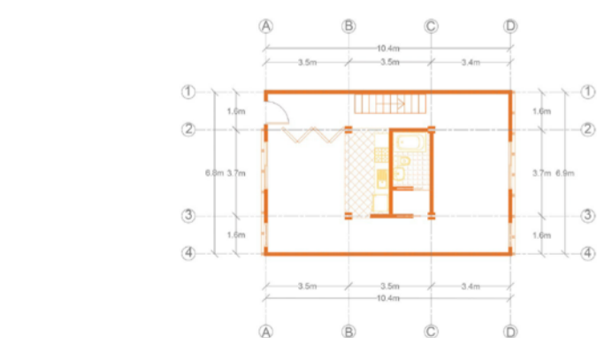
Planimetría barrial duplex 4. Escala 1:200.
