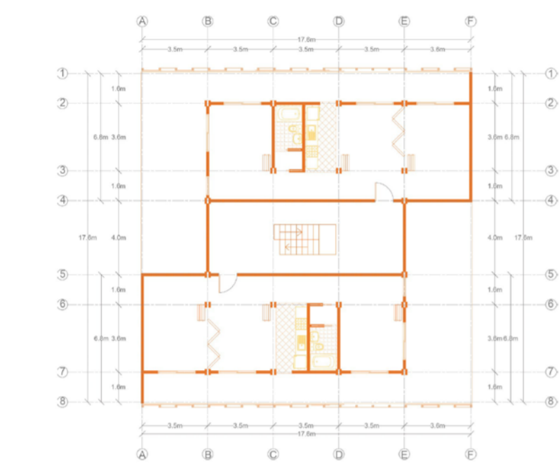
Planimetría barrial intermedia 2. Escala 1:200.
