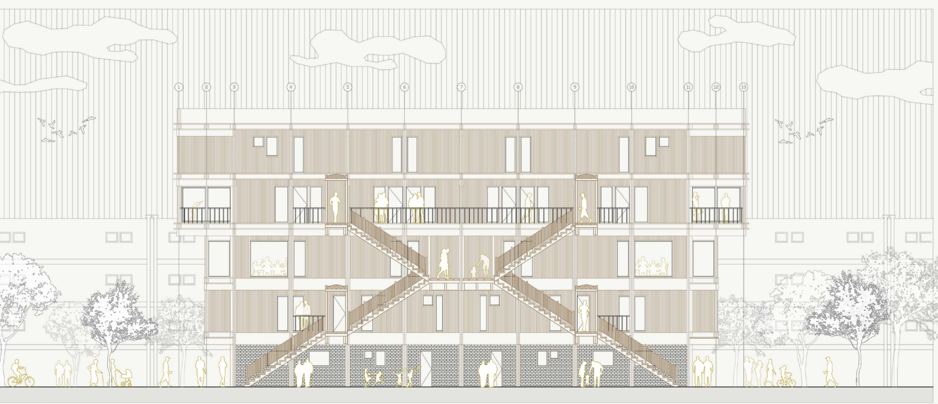
ELEVACIÓN LONGITUDINAL INTERIOR
