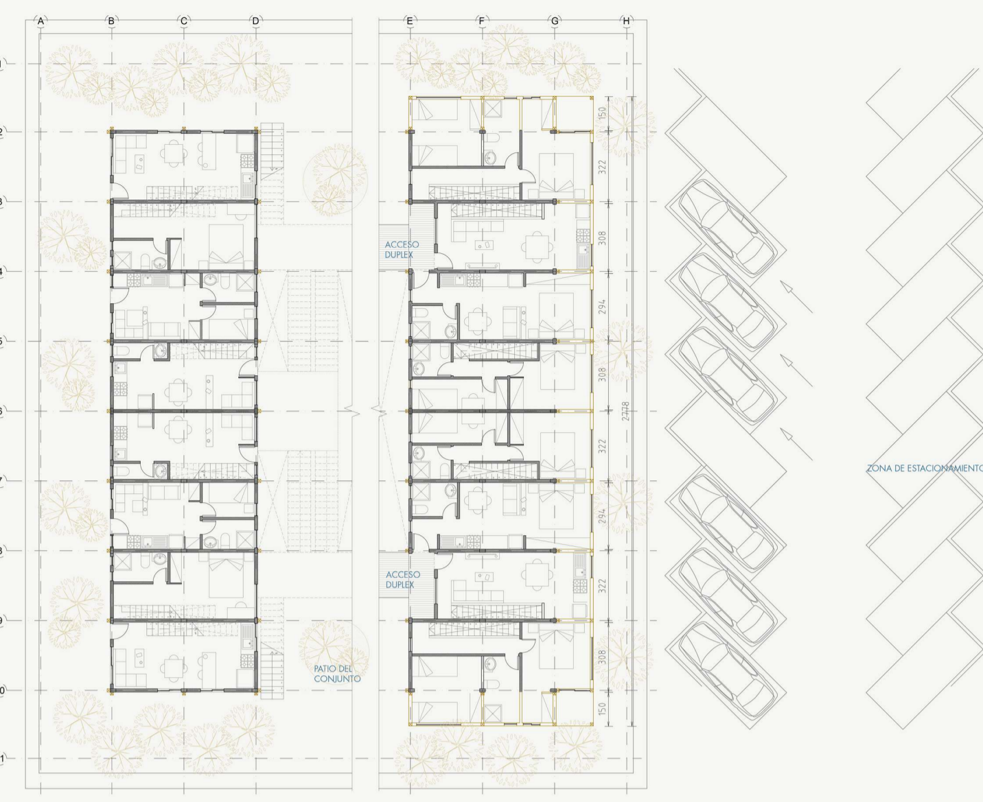
PLANTA PRIMER Y SEGUNDO PISO | ESTRUCTURA PREEXISTENTE | ESC. 1:175
