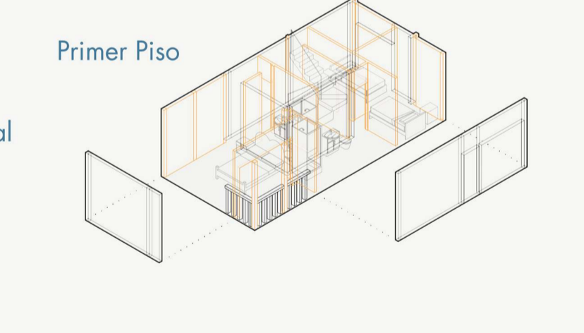
TIPOLOGÍA D Triplex Generacional (3 familias) 8D - 5B (151m2) esc. 1:75
