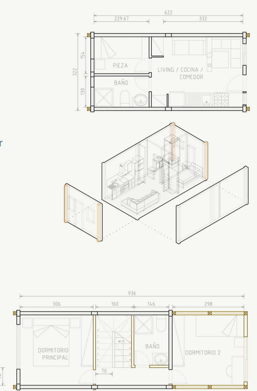
TIPOLOGÍA A (20m2) Pieza para arrendar esc. 1:75
