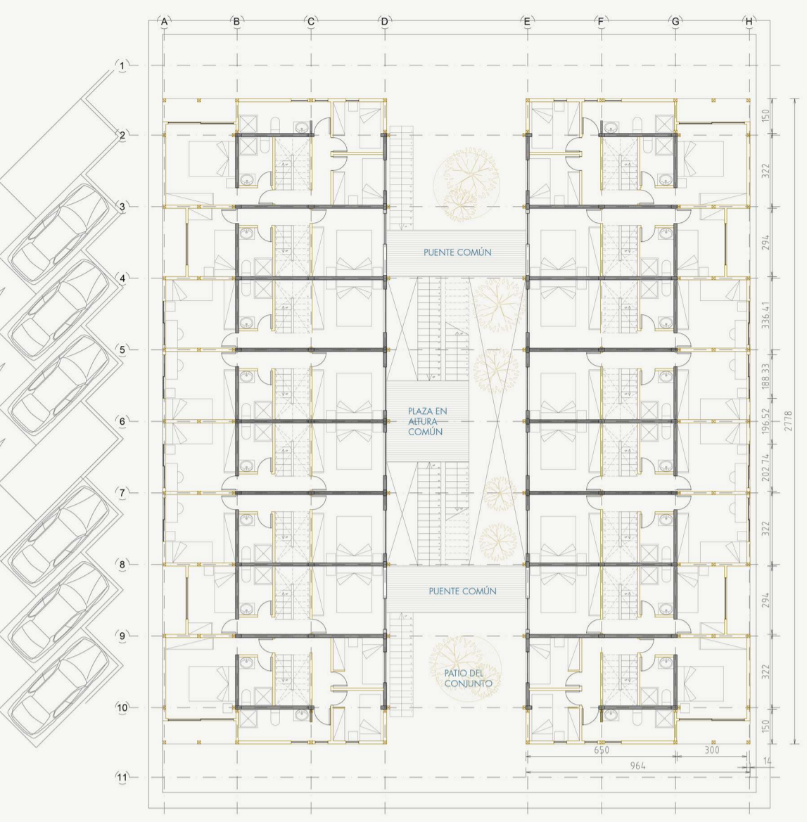
PLANTA TERCER PISO | ESTRUCTURA PREEXISTENTE Y KOALA | ESC. 1:175
