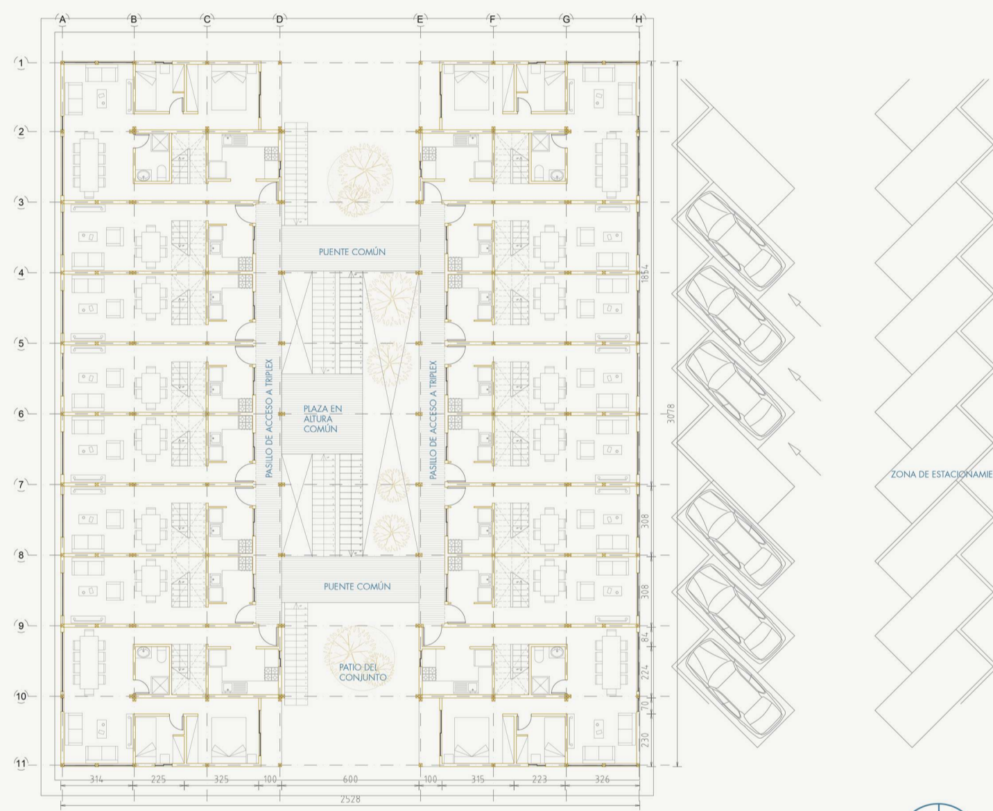
PLANTA CUARTI PISO | ESTRUCTURA KOALA | ESC. 1:175
