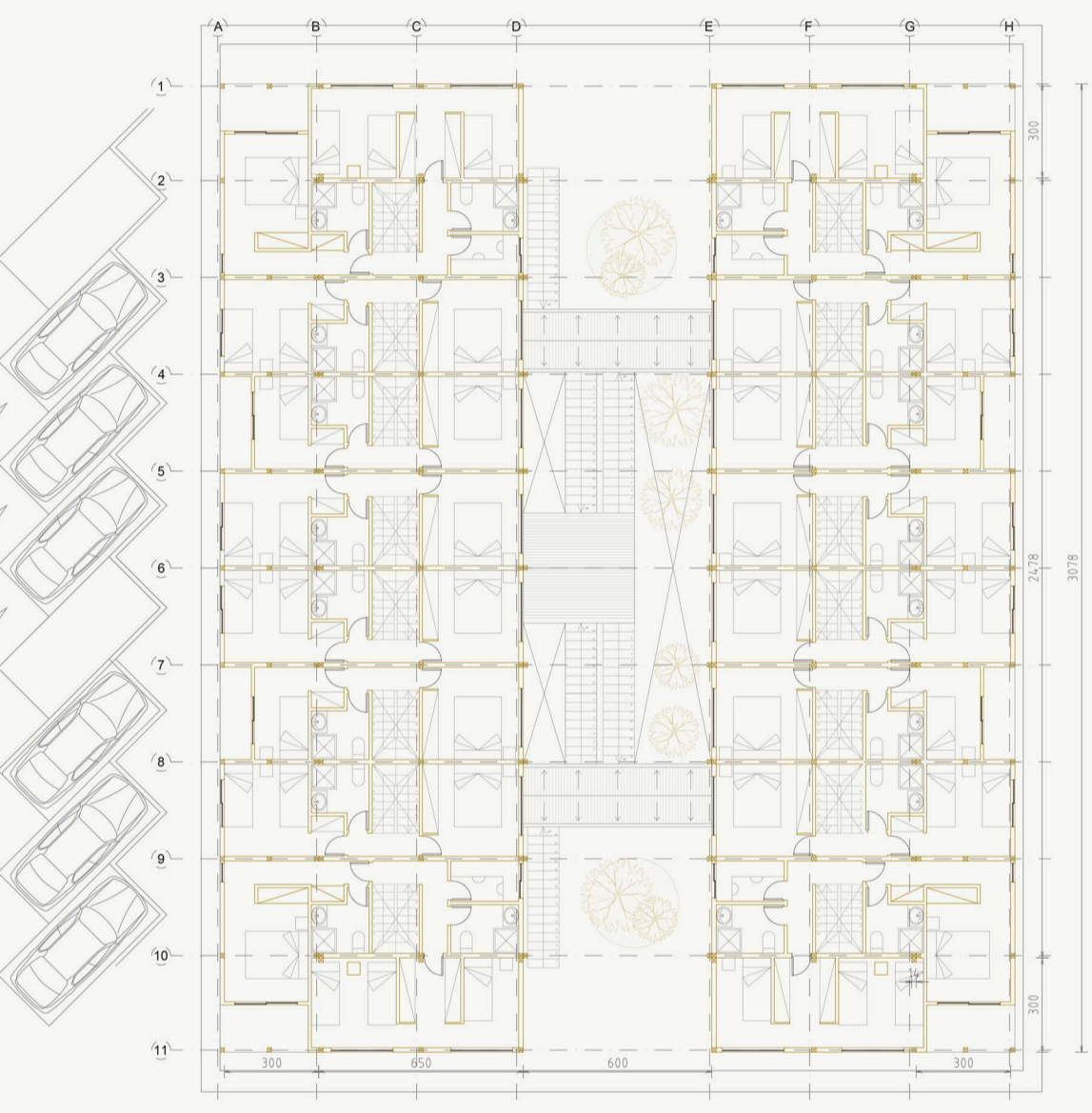
PLANTA QUINTO PISO | ESTRUCTURA KOALA | ESC. 1:175
