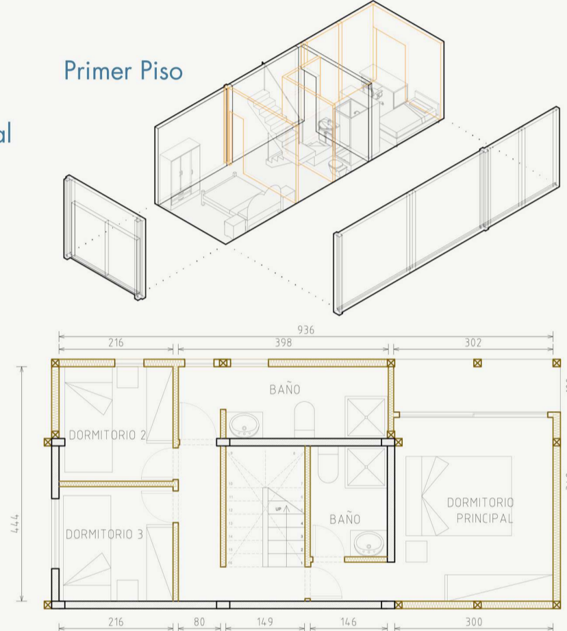
TIPOLOGÍA C Triplex Generacional (2 familias) 4D - 2B (87m2) esc. 1:75
