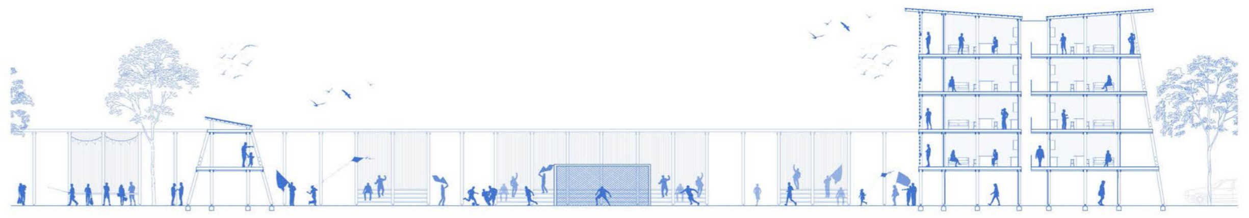
CORTE A-A' 1:250
