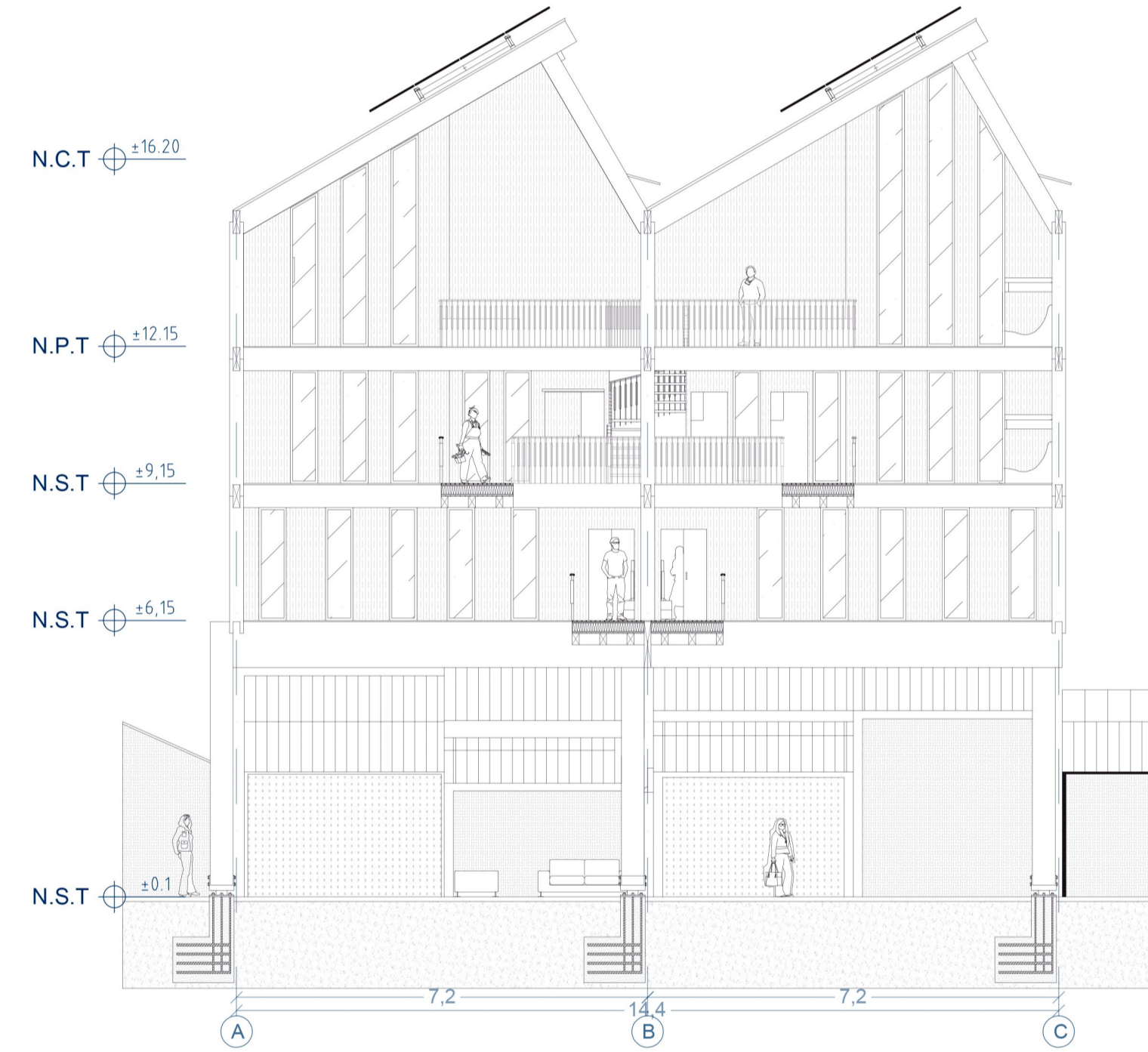
CORTE A´A´ ESC.:1:125
