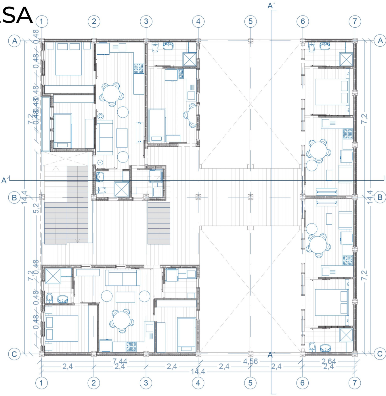
PLANTA NIVEL 1 SOBRE-MESA ESC:1:125
