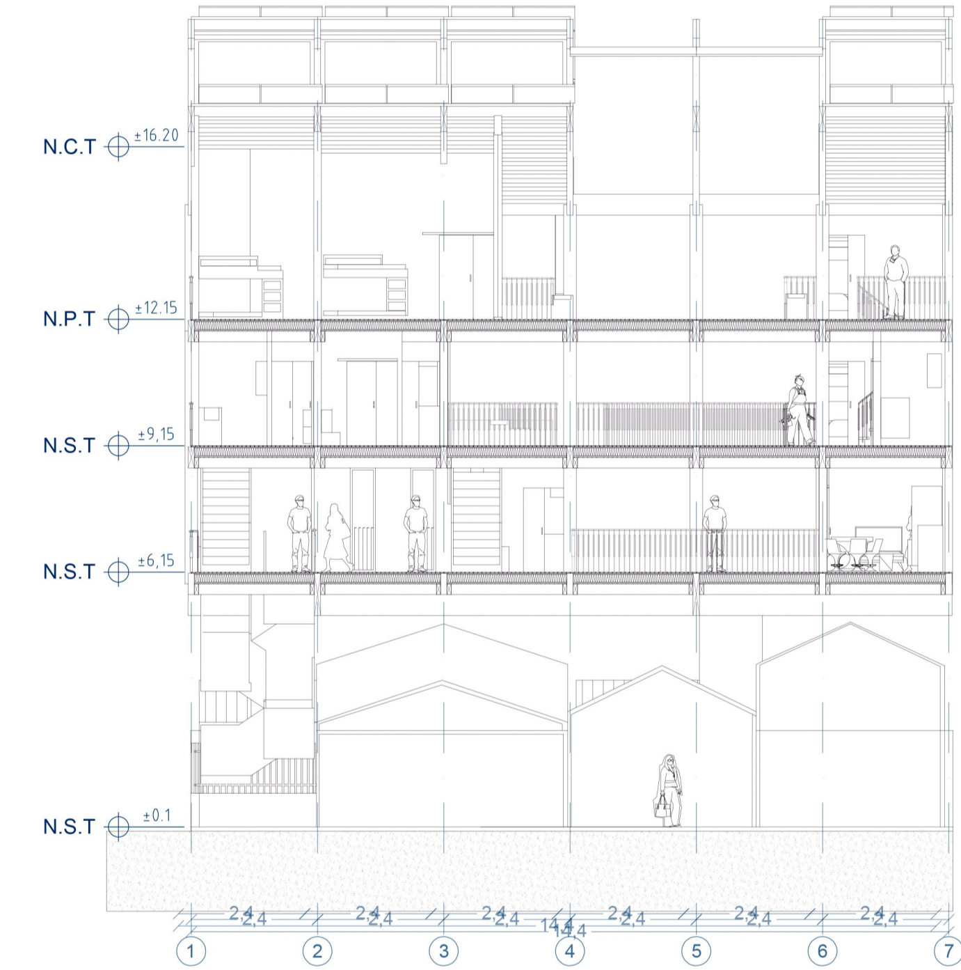
CORTE B´B´ ESC.:1:125
