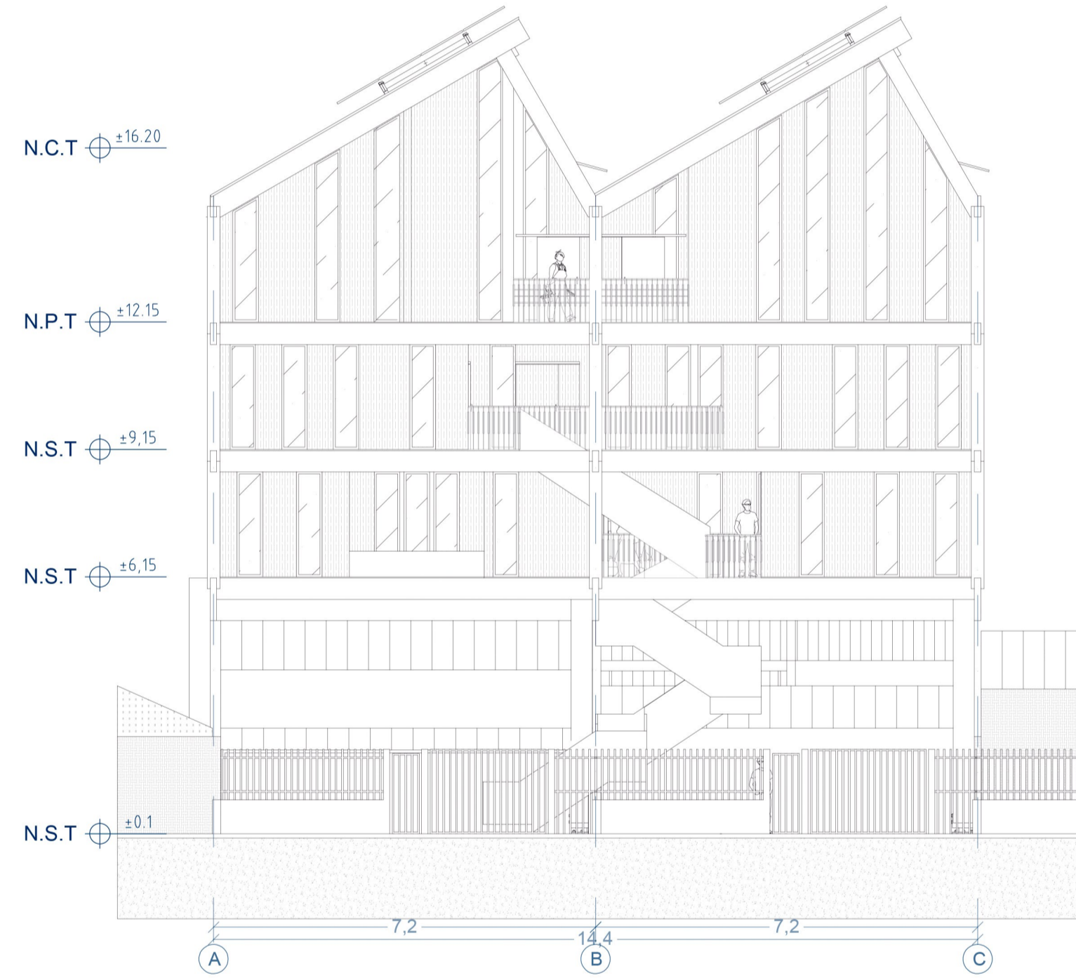
ELEVACIÓN OESTE ESC.:1:125
