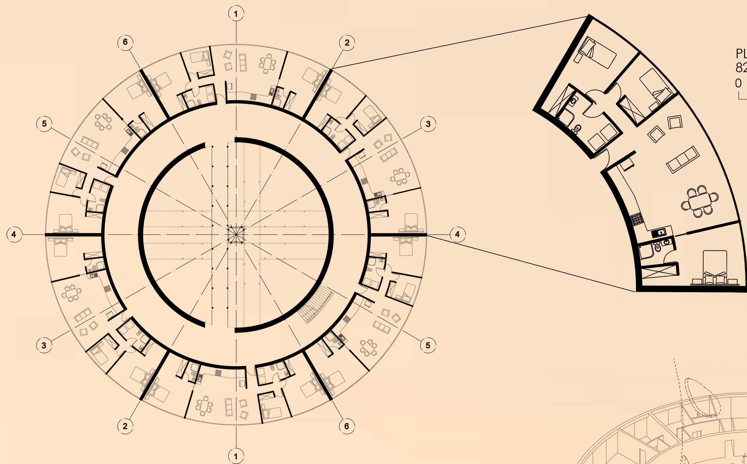
PLANTA PISO 11 0 5 10
