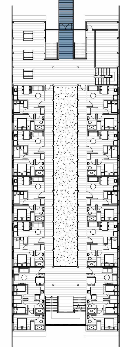
Planta nivel 3 / esc. 1:350
