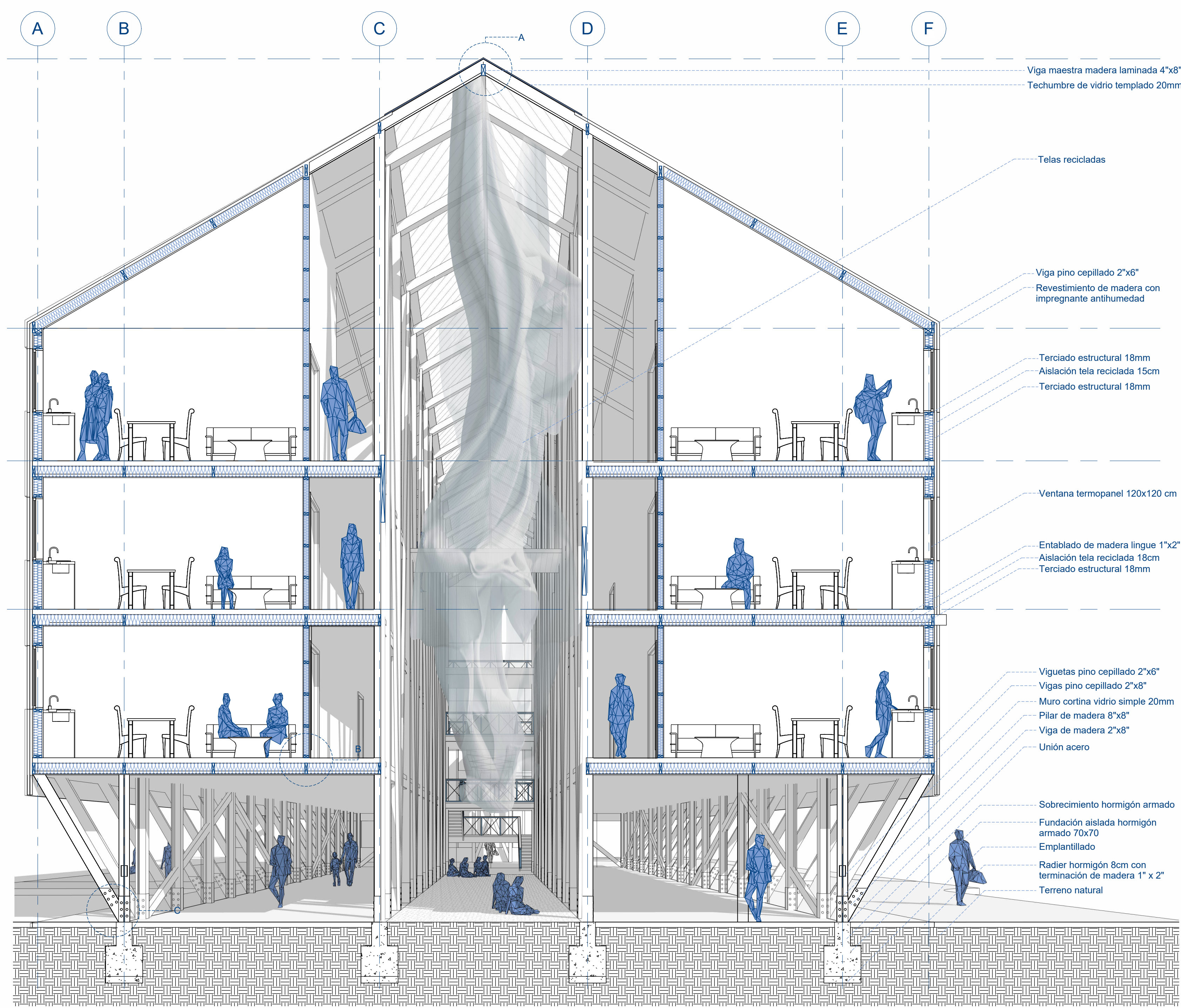
Corte constructivo / esc. 1:50
