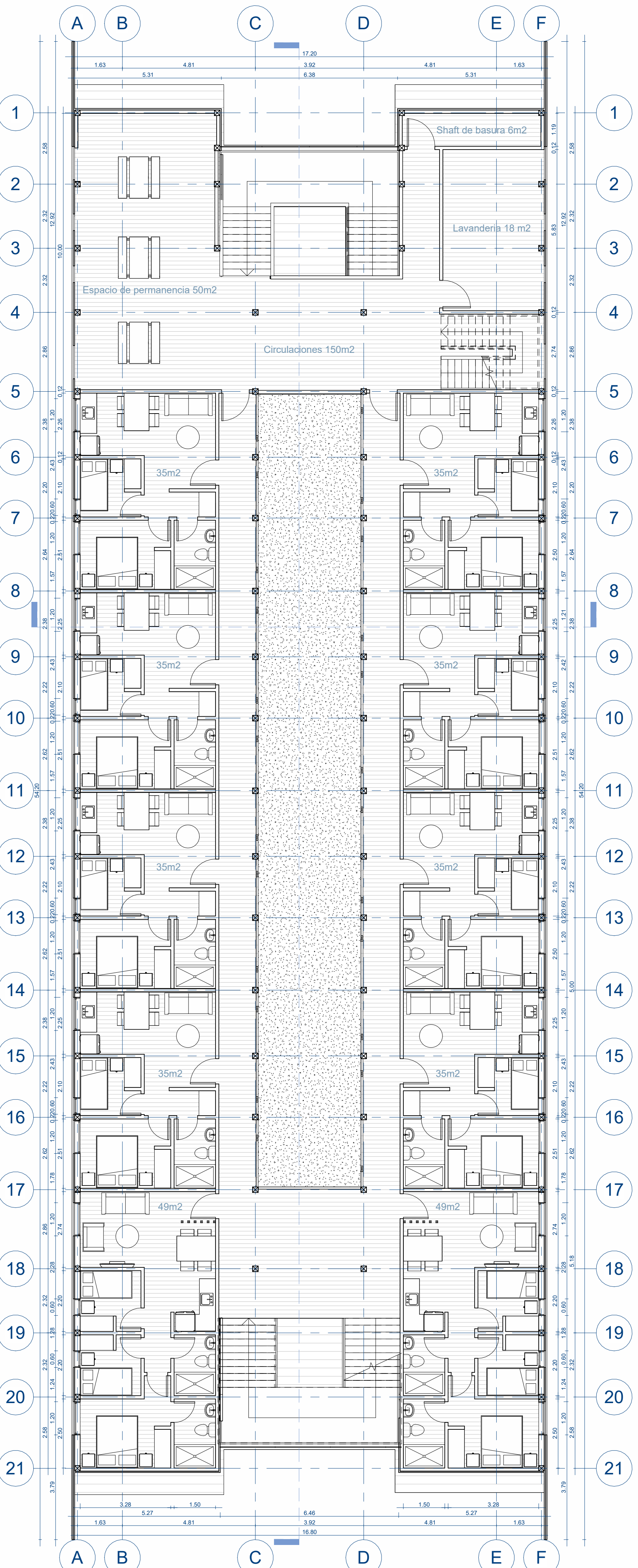
Planta tipo nivel 2 / esc. 1:100
