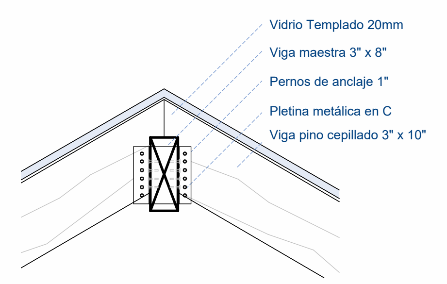
Detalle constructivo A / esc. 1:10
