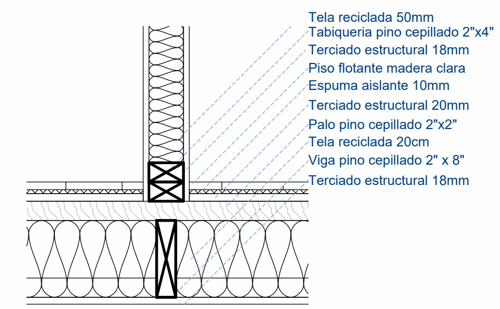
Detalle constructivo B / esc. 1:10
