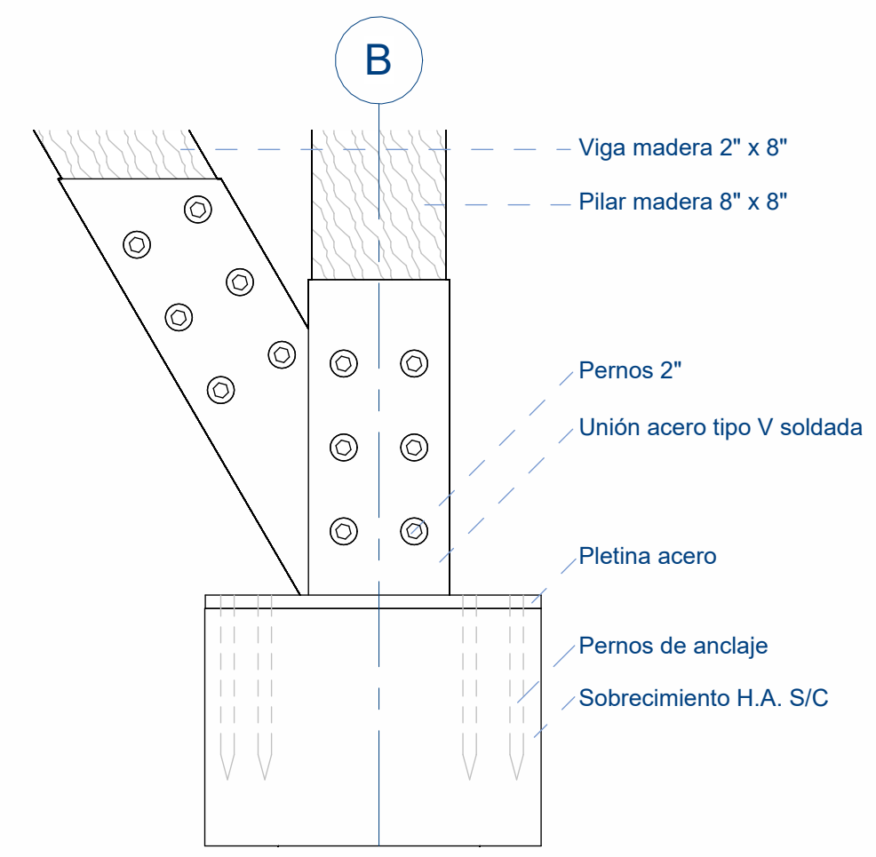
Detalle constructivo C / esc. 1:10
