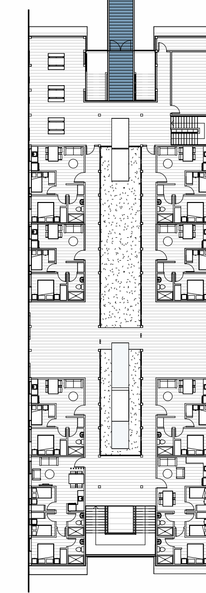
Planta nivel 4 / esc. 1:350
