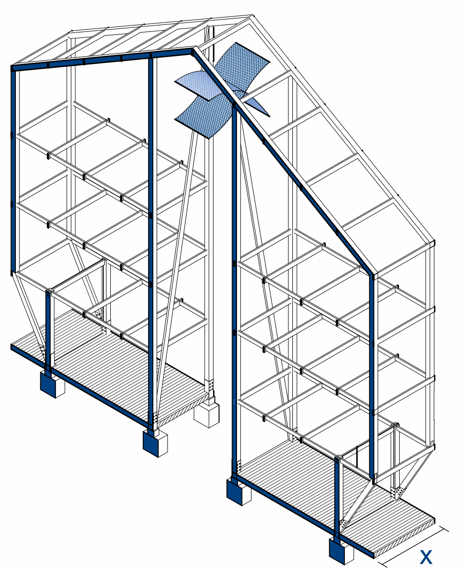
Estructura modular / x seg. recinto esc. 1:150
