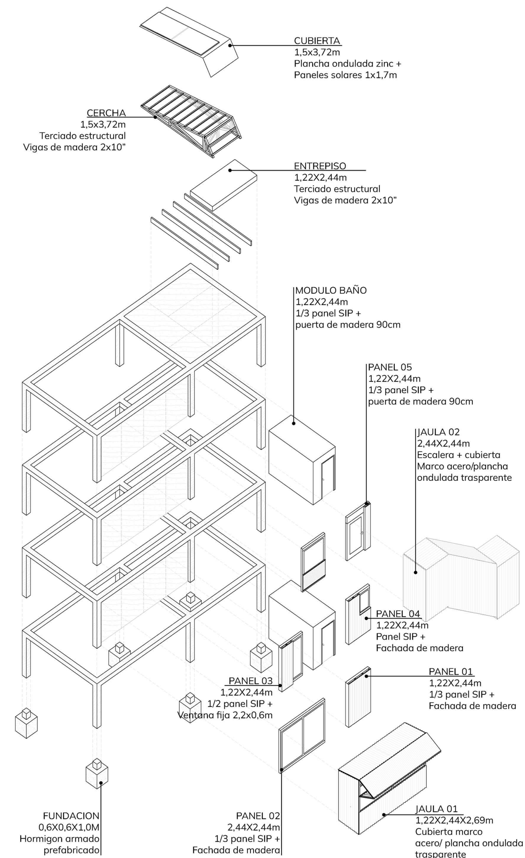
Explotado isometrico
