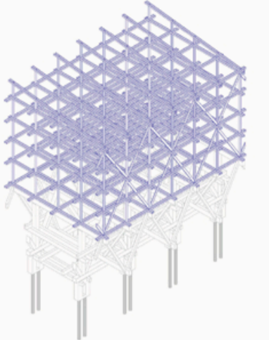
USO DE GRILLA SISTEMA DOBLE VIGA
