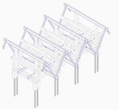
CABALLETE INVERTIDO RECUPERACIÓN DE LÓGICA ESTRUCTURAL
