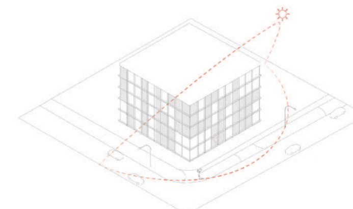
CONTROL LUMÍNICO
