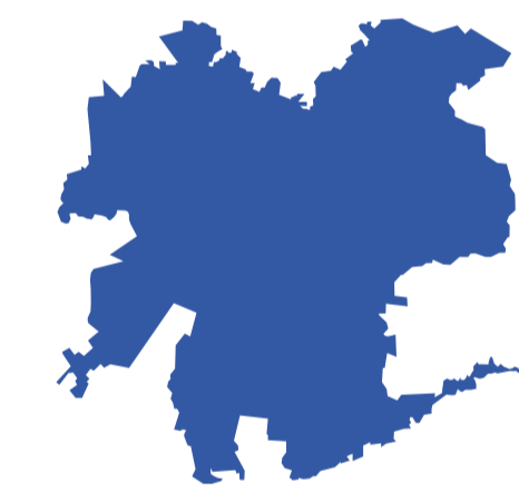
Region Metropolitana
