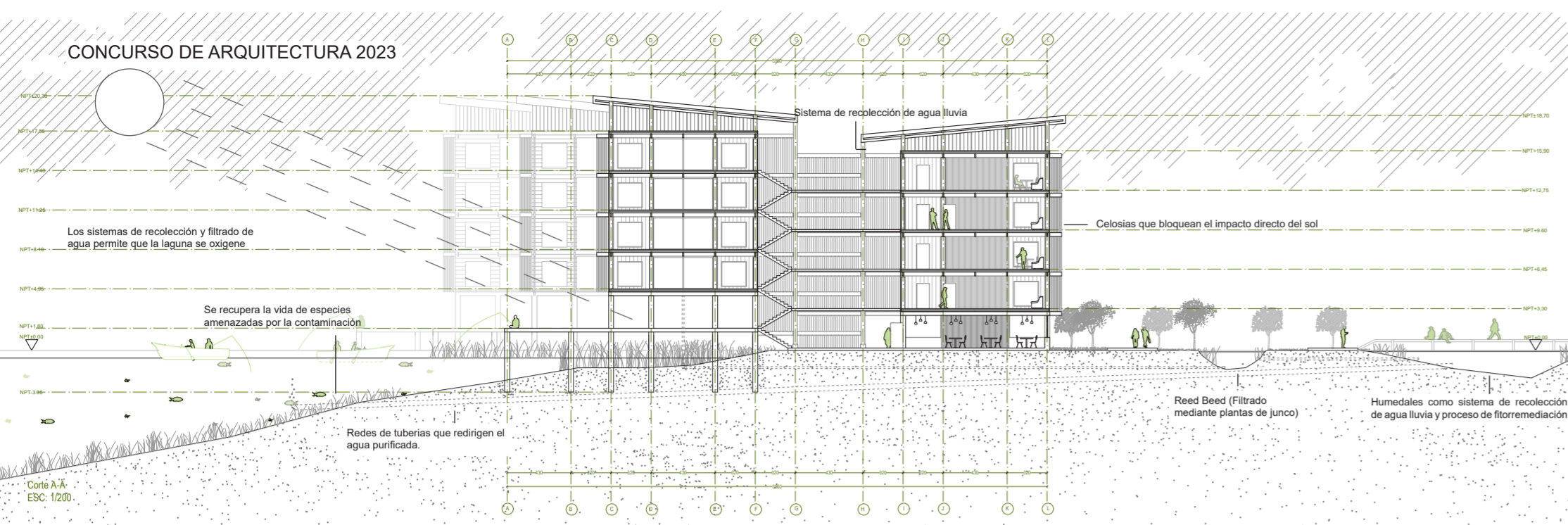
CORTE ESC 1:400
