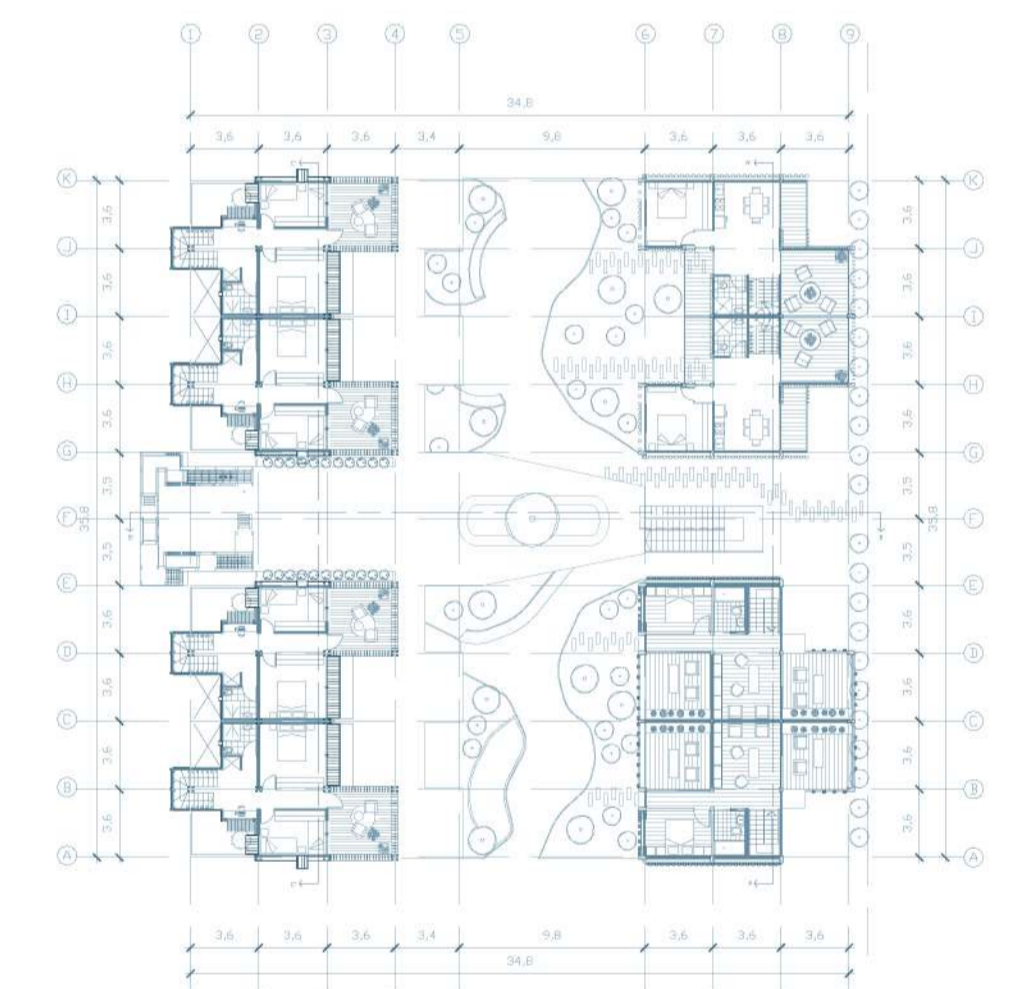
PLANTA CONJUNTO TERCER NIVEL
