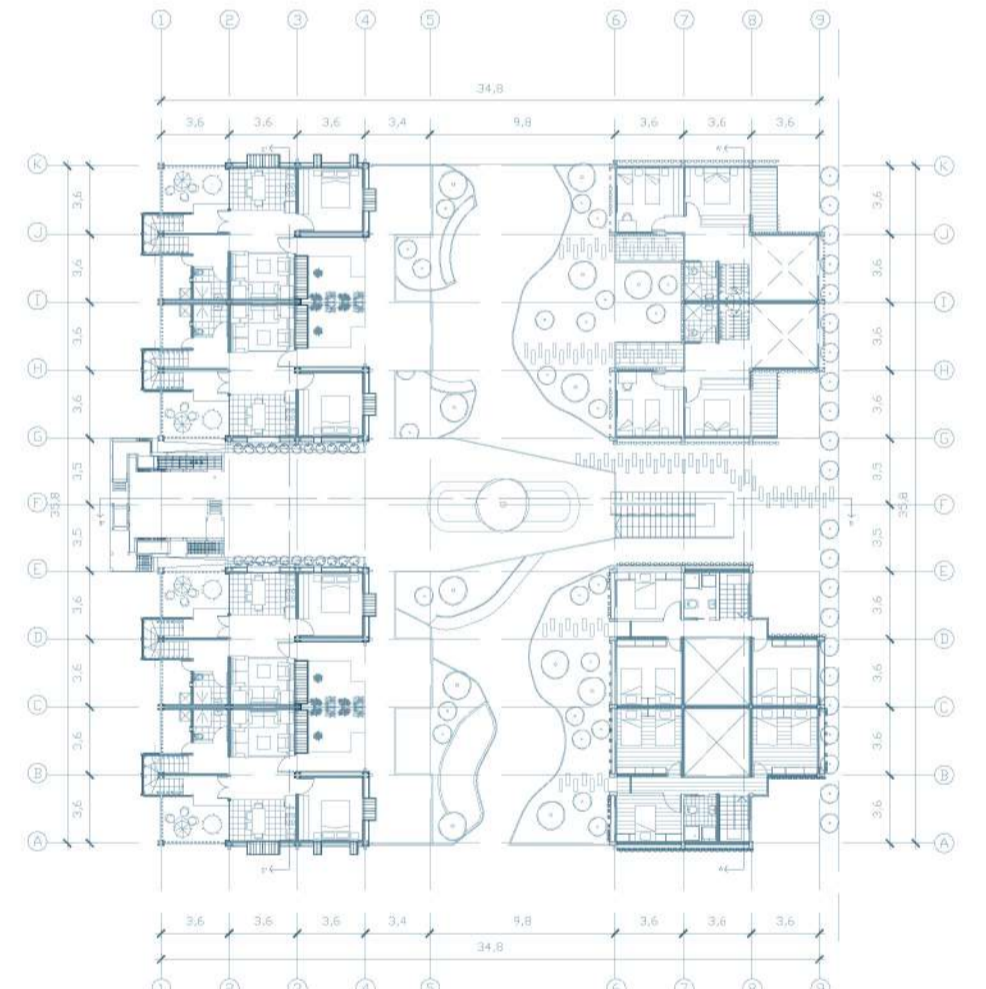
PLANTA CONJUNTO SEGUNDO NIVEL
