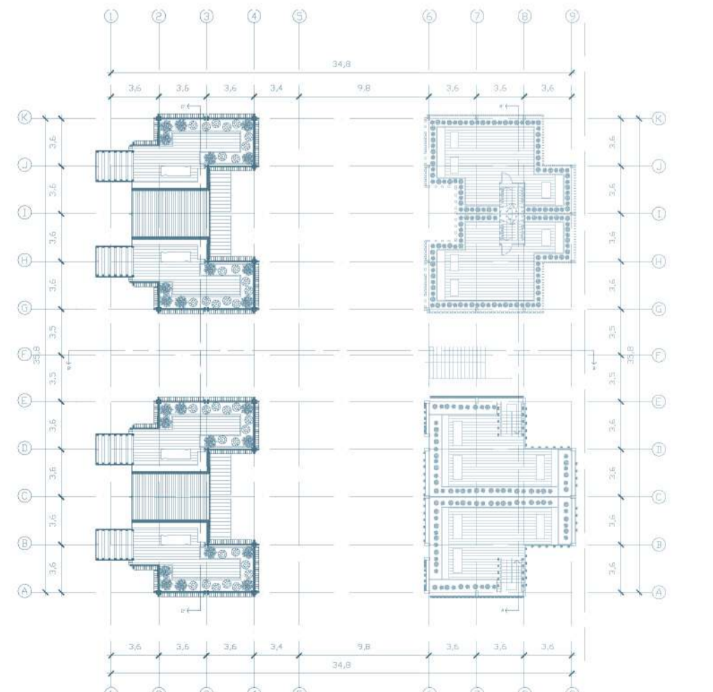
PLANTA CONJUNTO QUINTO NIVEL
