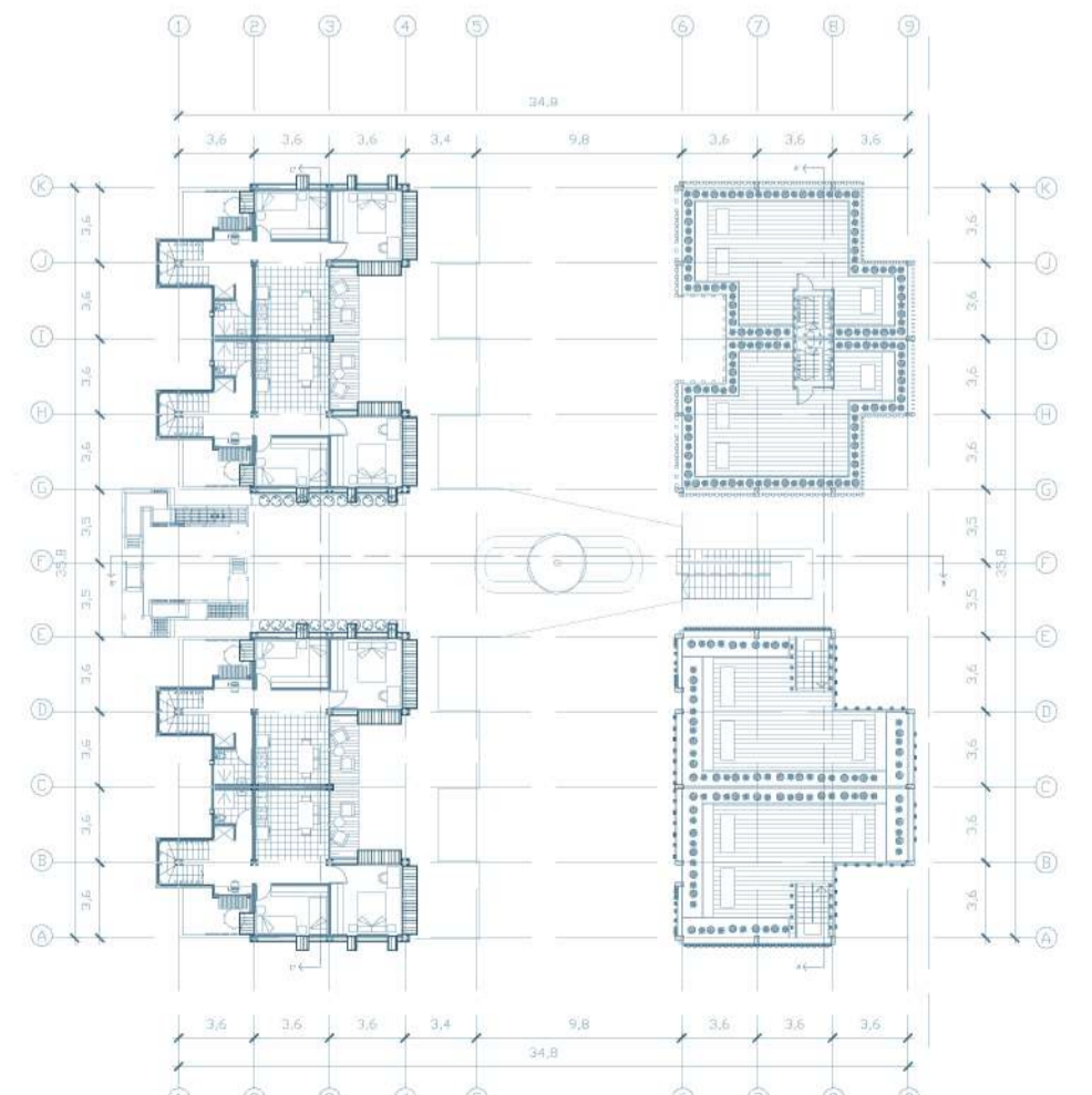
PLANTA CONJUNTO CUARTO NIVEL
