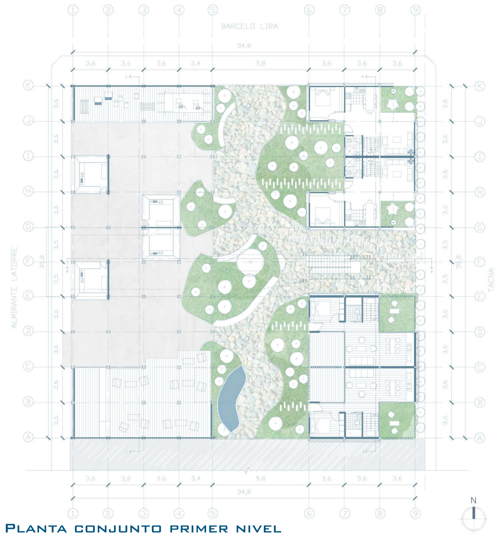
PLANTA CONJUNTO PRIMER NIVEL
