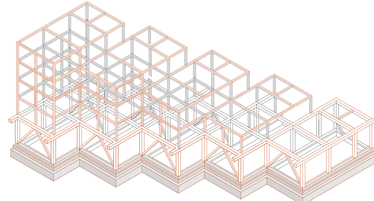
ENTRAMADO DE MADERA VIVIENDAS
