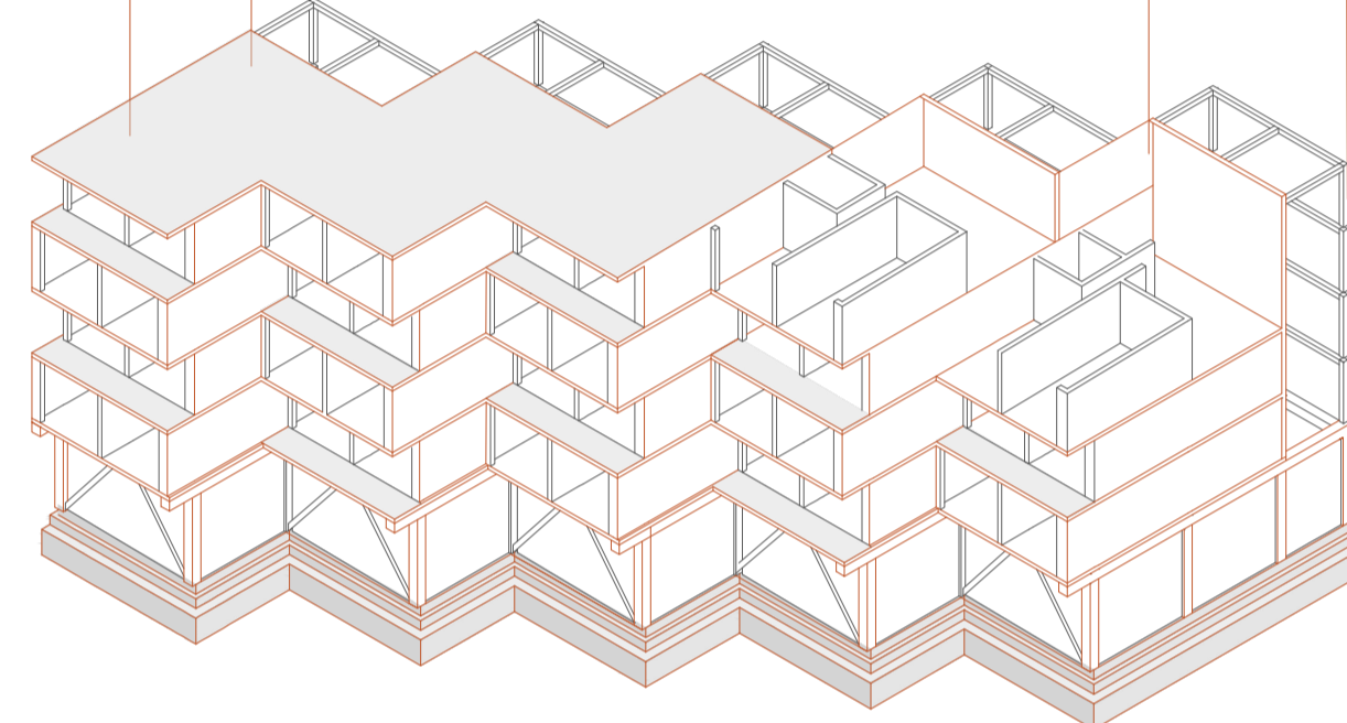
SUELO, TECHO Y MUROS ESTRUCTURALES DE CLT
