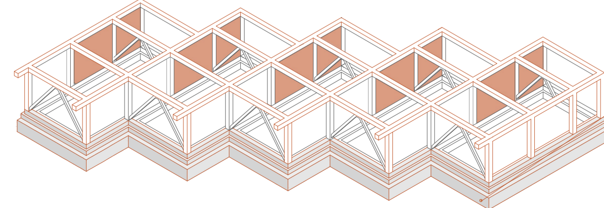
ENTRAMADO PORTANTE DE MADERA, ARRIOSTAMIENTO, FUNDACIONES HAY MUROS ESTRUCTURALES CLT
