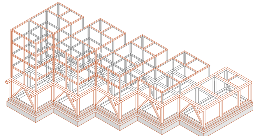
ENTRAMADO PORTANTE DE MADERA, ARRIOSTAMIENTO, FUNDACIONES HAY MUROS ESTRUCTURALES CLT
