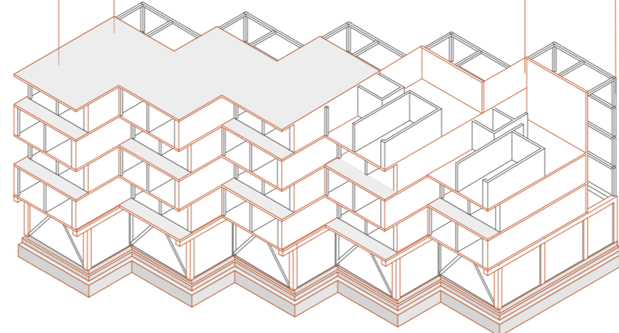
SUELO, TECHO Y MUROS ESTRUCTURALES DE CLT
