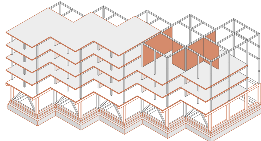
ENTRAMADO DE MADERA VIVIENDAS
