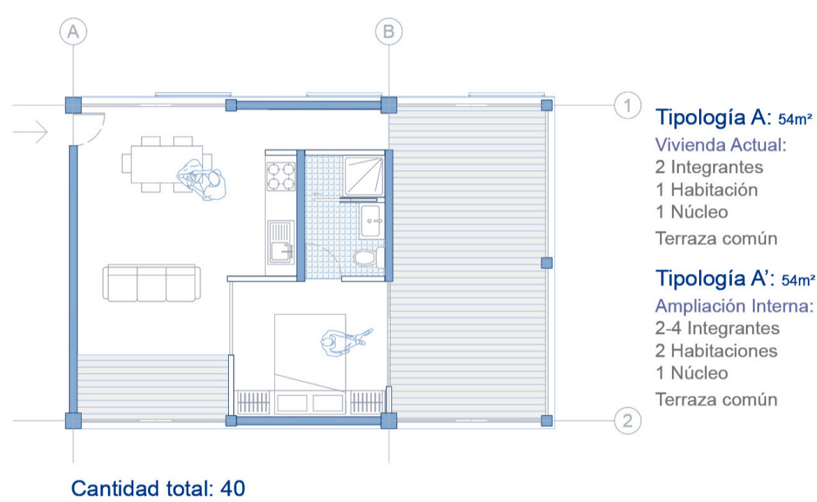
TIPOLOGÍAS / Esc. 1:100
