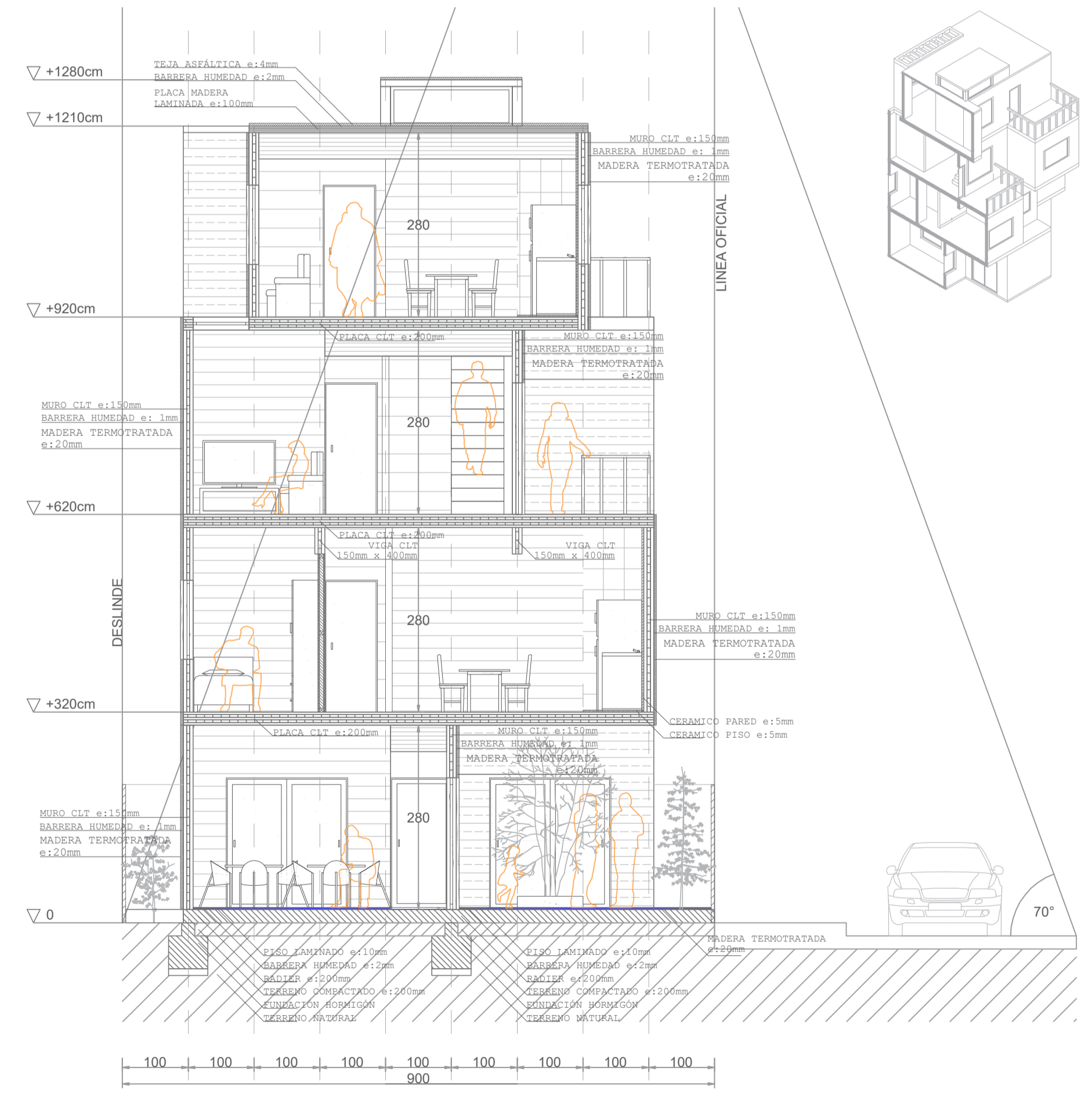
Corte B-B'
