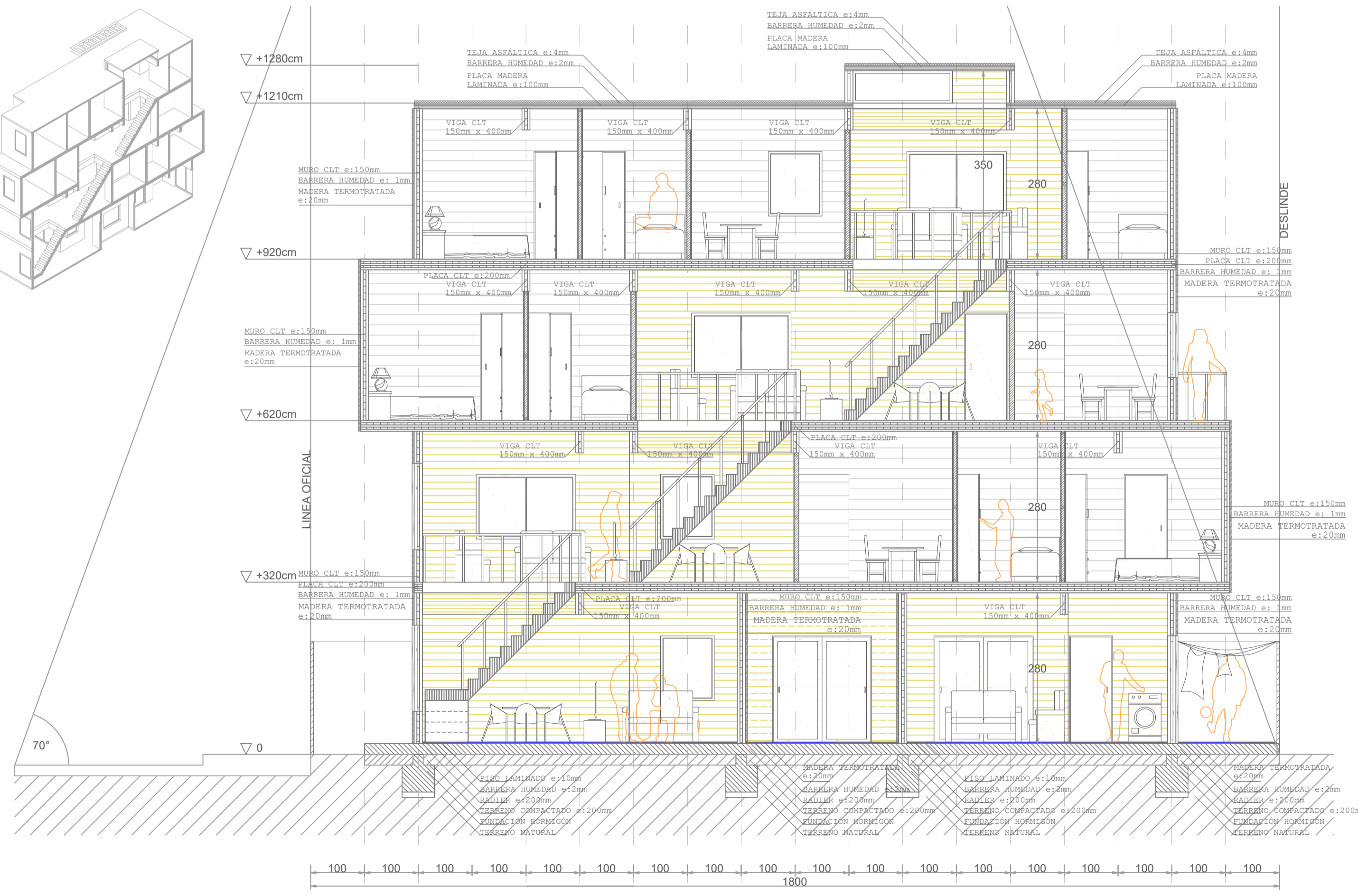
Corte A-A'
