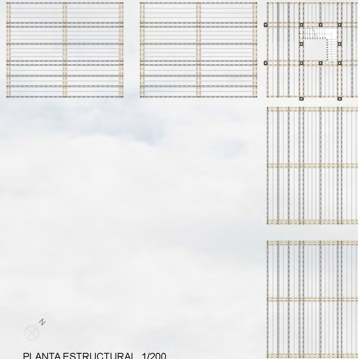
PLANTA ESTRUCTURAL 1/200
