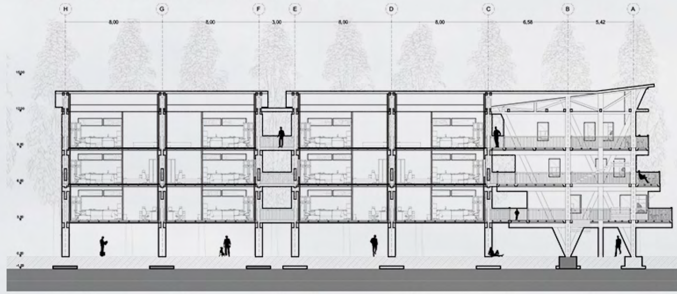
SECCIONES LONGITUDINALES 1/200
