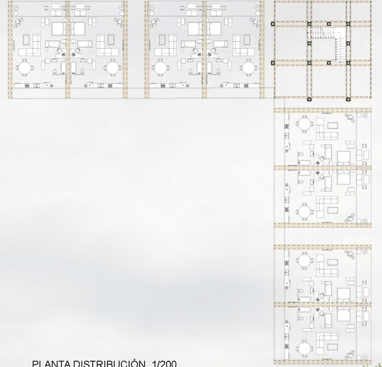
PLANTA DISTRIBUCIÓN 1/200
