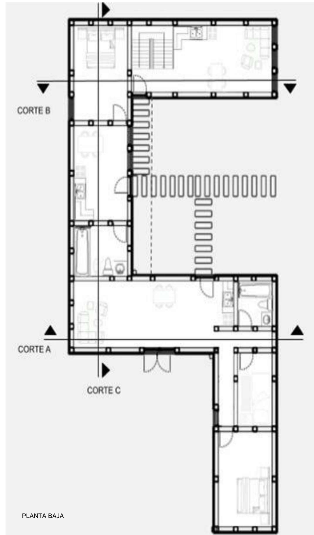
PLANTAS
