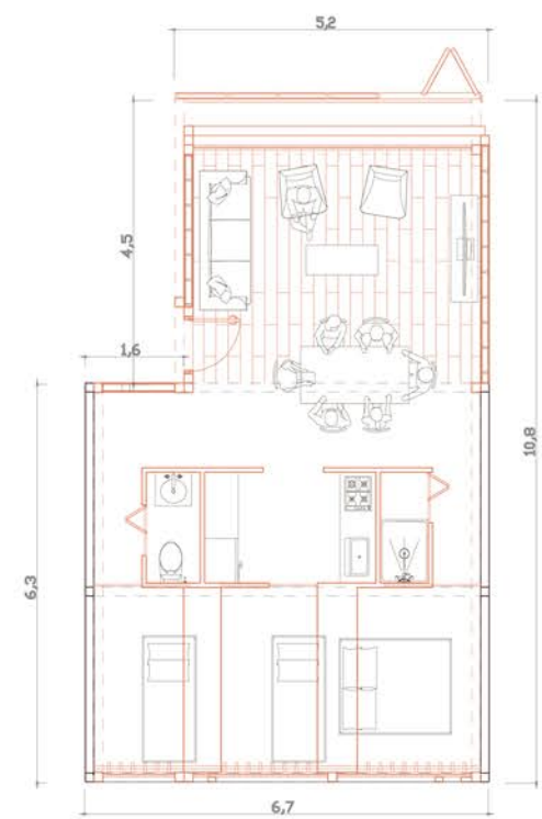
PLANTA DEPARTAMENTO GRANDE 66 m 2 ESC 1:50
