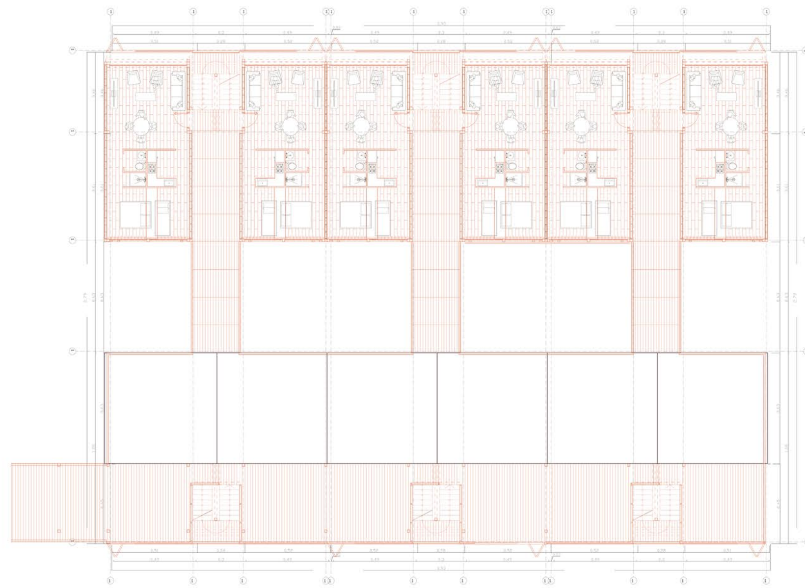
PLANTA TERCER PISO (NIVEL TERRAZA) ESC 1: 100
