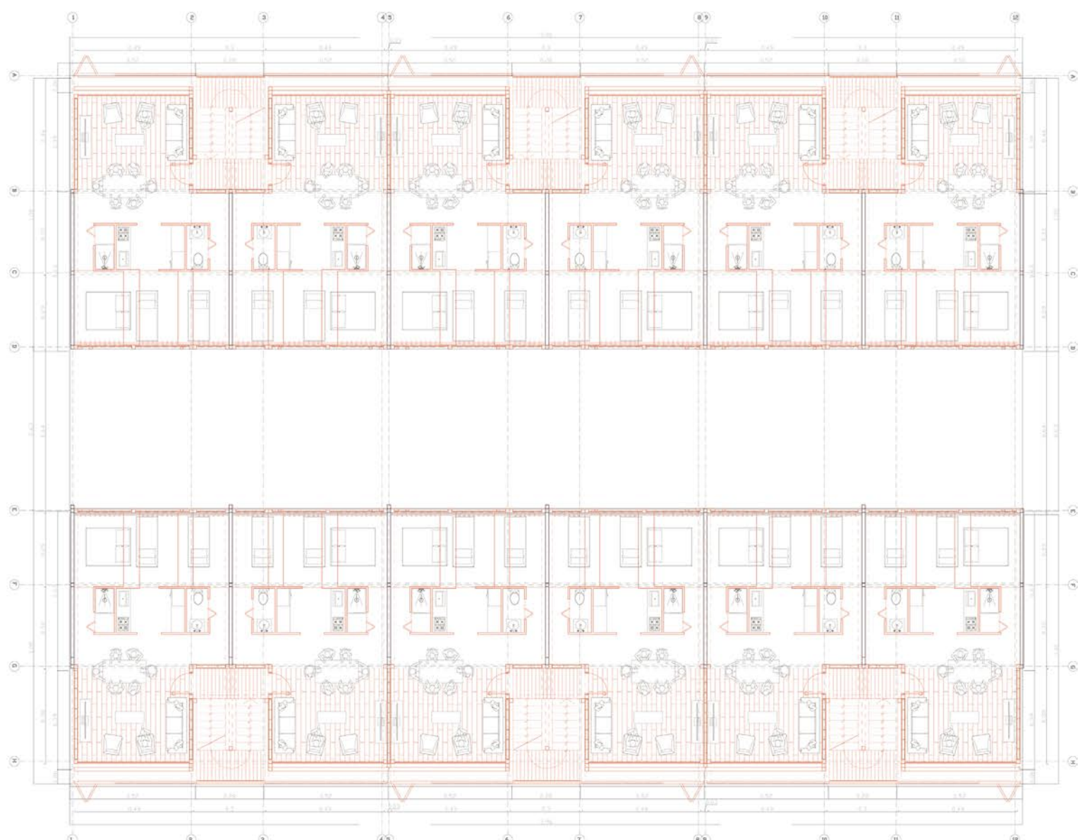
PLANTA PRIMER PISO (NIVEL CALLE) ESC 1: 100
