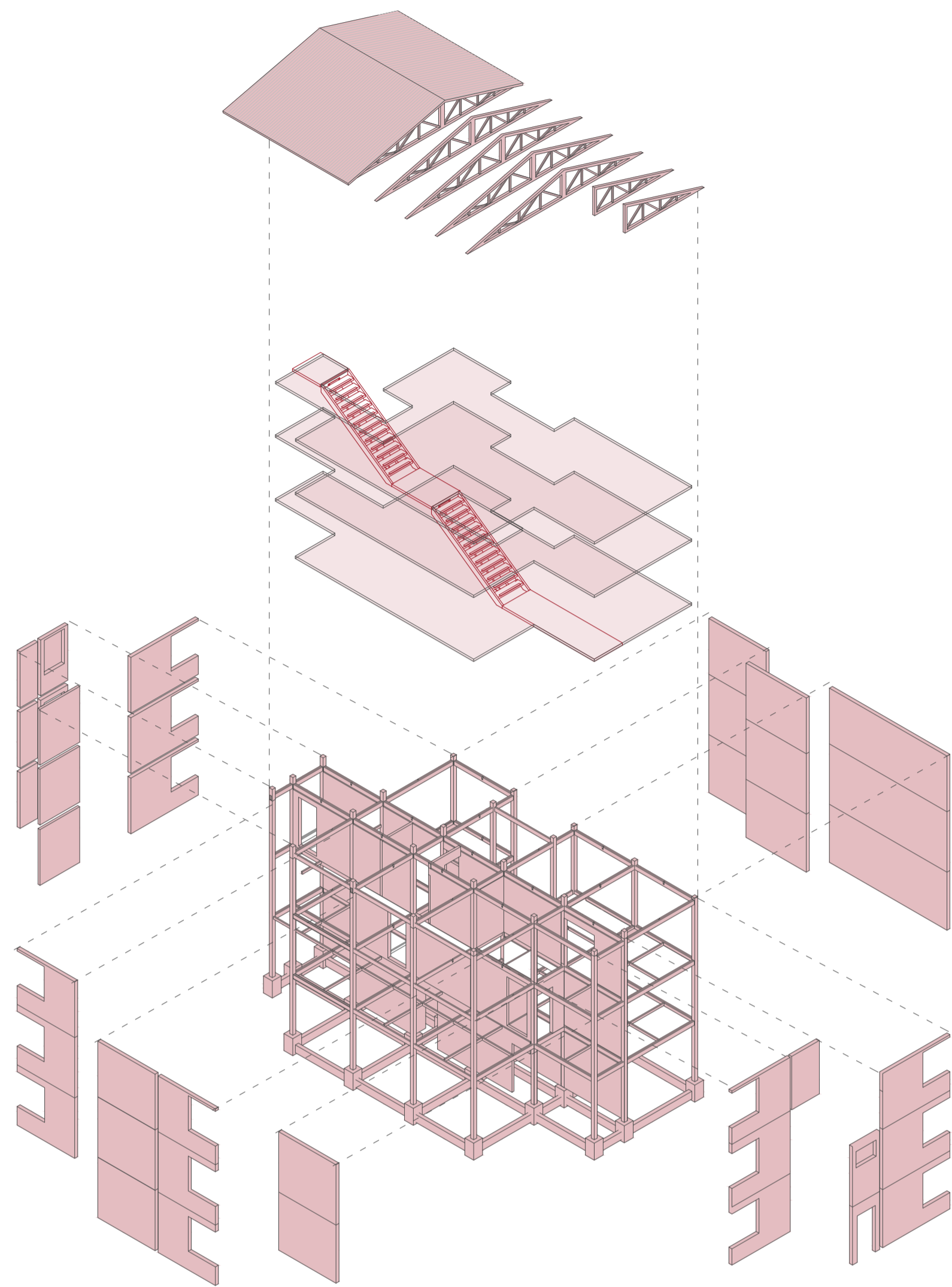
Isometrica Estructural 1:100
