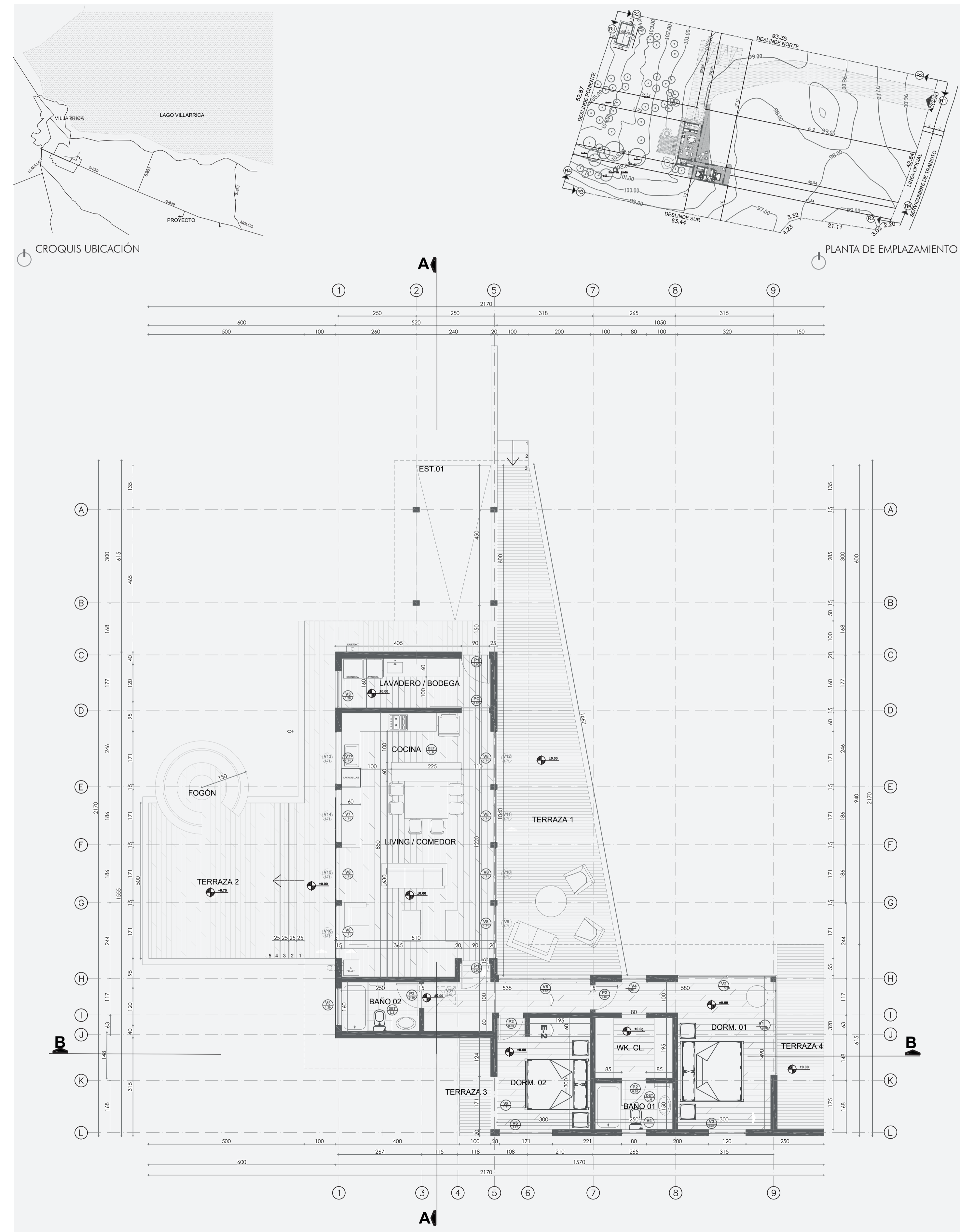
PLANTA DE ARQUITECTURA ESCALA 1:50
