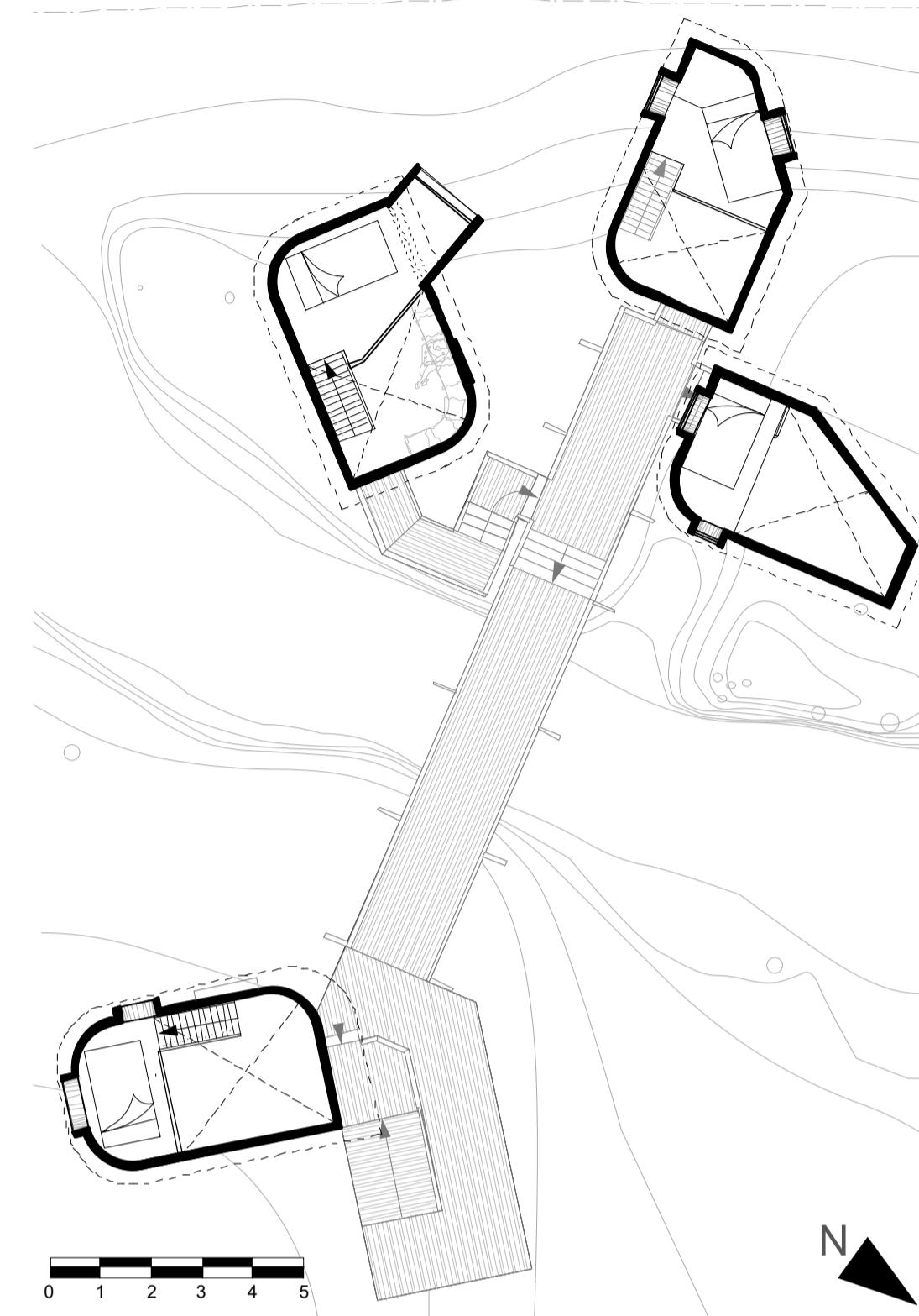
PLANTA CONJUNTO 2DO NIVEL
