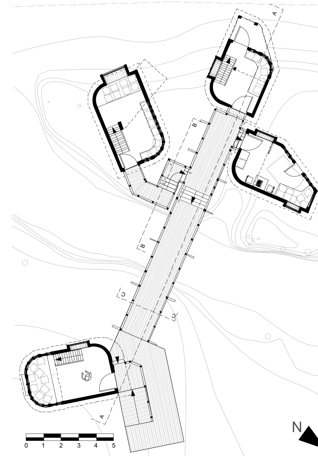
PLANTA CONJUNTO 1ER NIVEL
