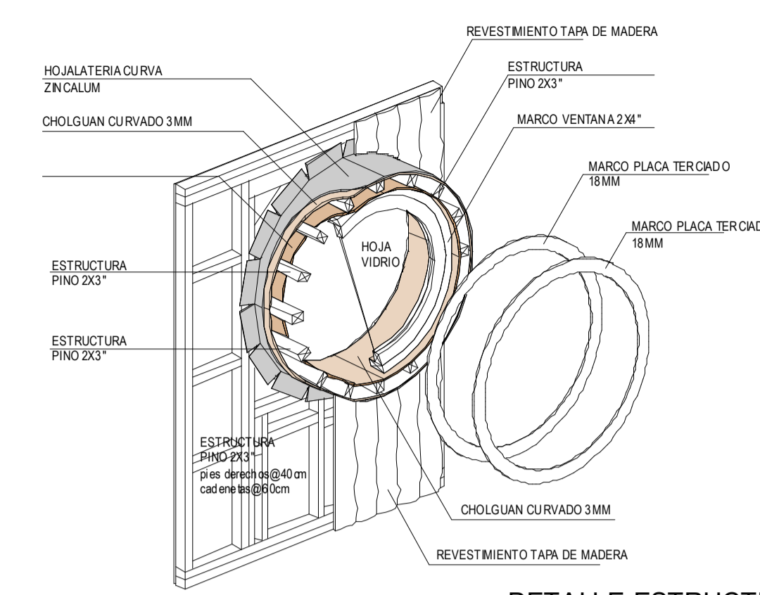
DETALLE ESTRUCTURA GENERICA BOWINDOWS
