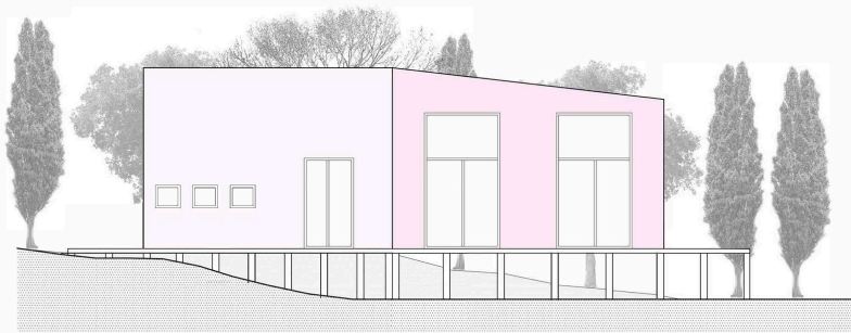
ELEVACIÓN NORORIENTE
