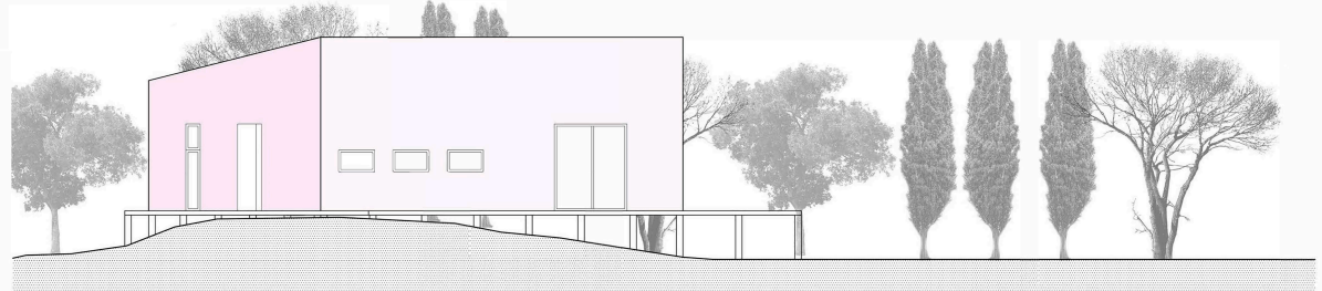
ELEVACIÓN SURORIENTE
