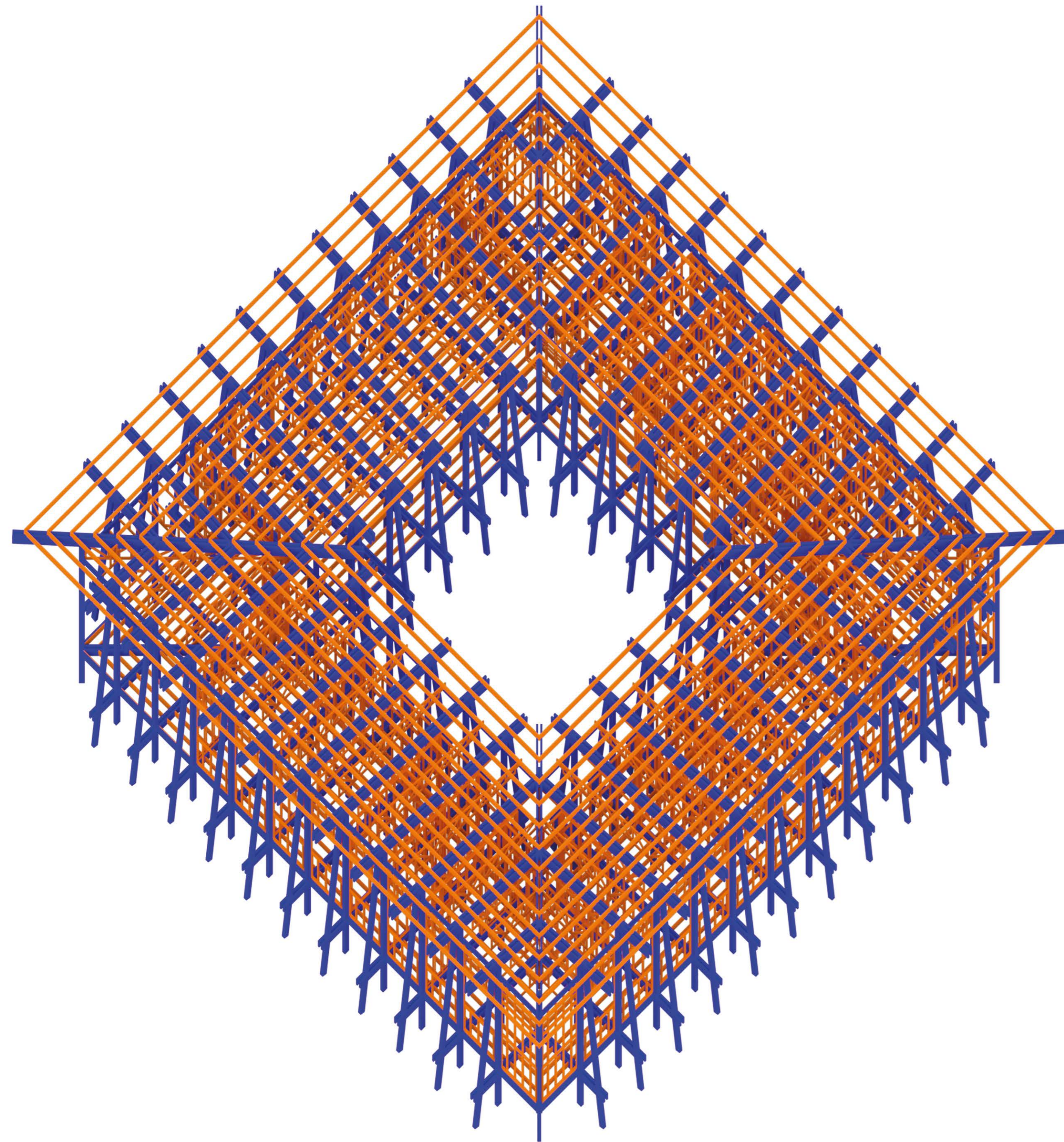
Axonometrica de elementos prefabricados y mecanizados de madera
