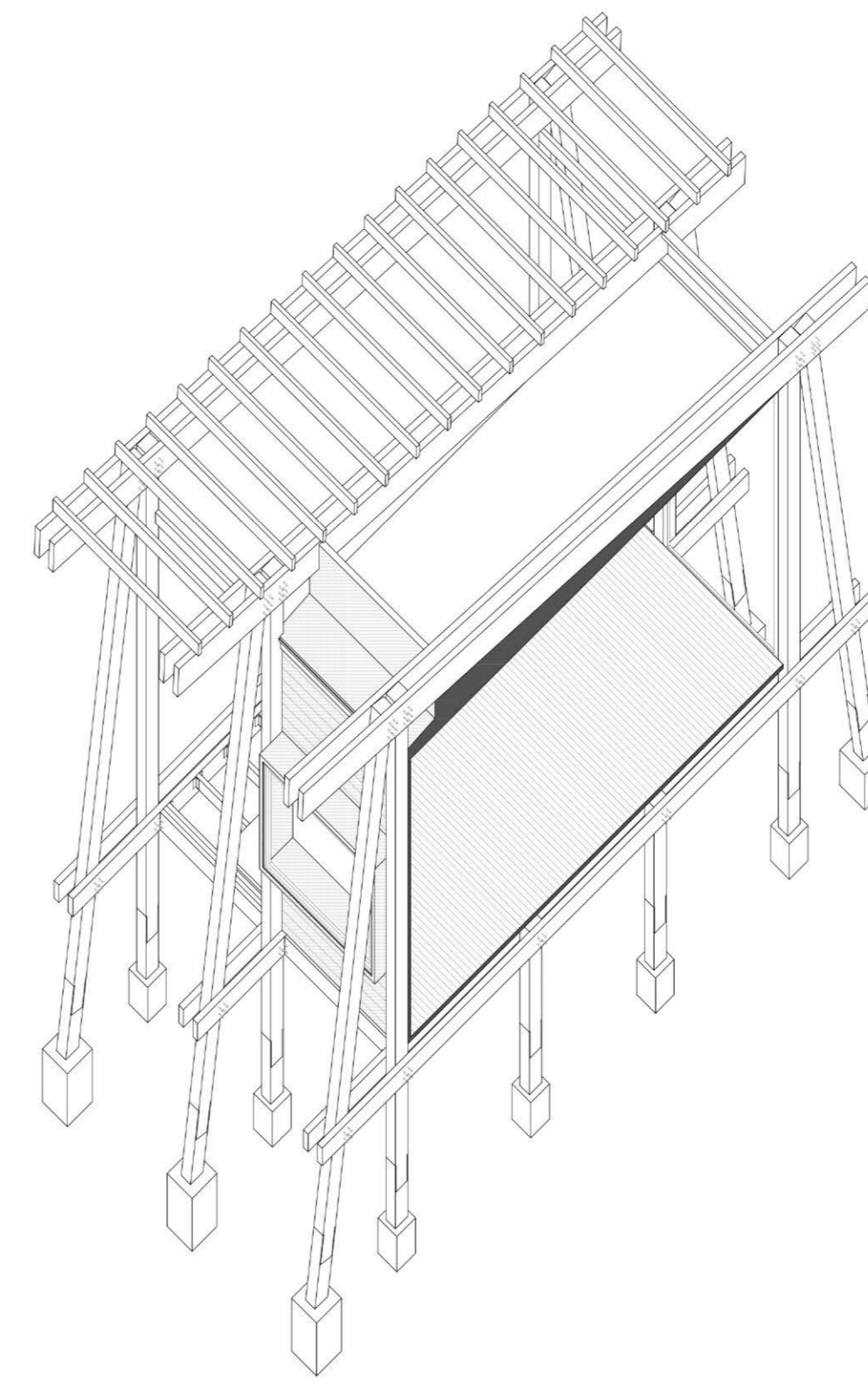
Axonometrica Detalle
