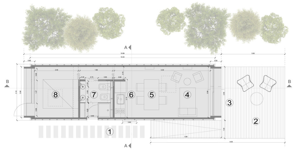
PLANTA (Sup. Cubierta: 30m 2 )
