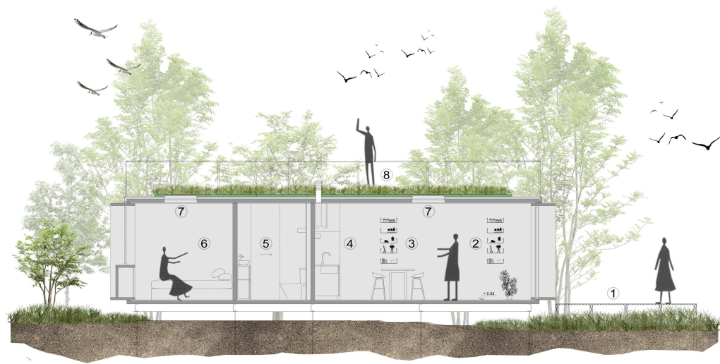
CORTE B
