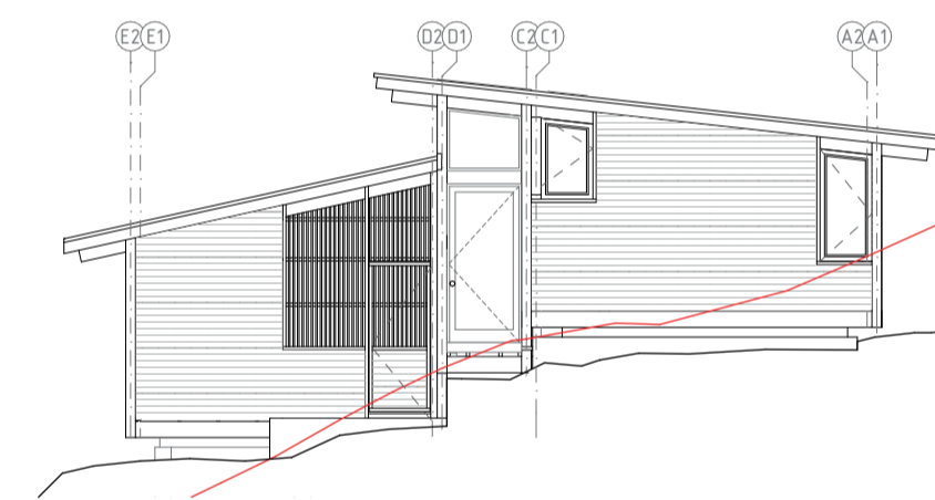
Elevación Oriente 0 50 100 200
