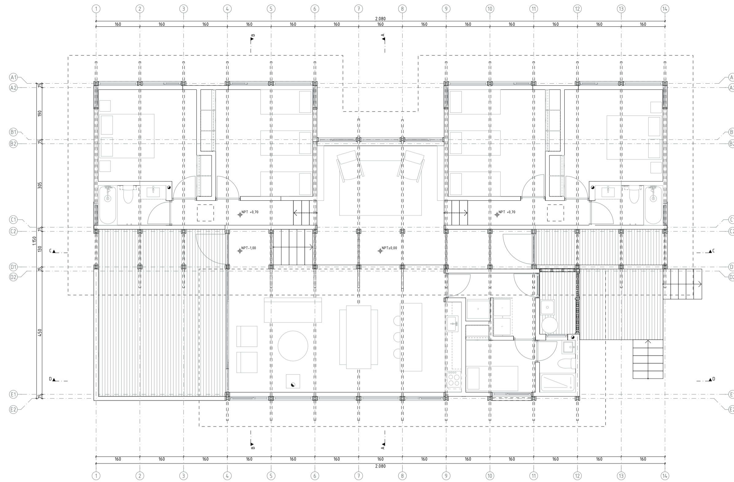
Planta 0 50 100 200
