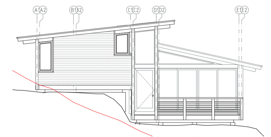
Elevación Poniente 0 50 100 200
