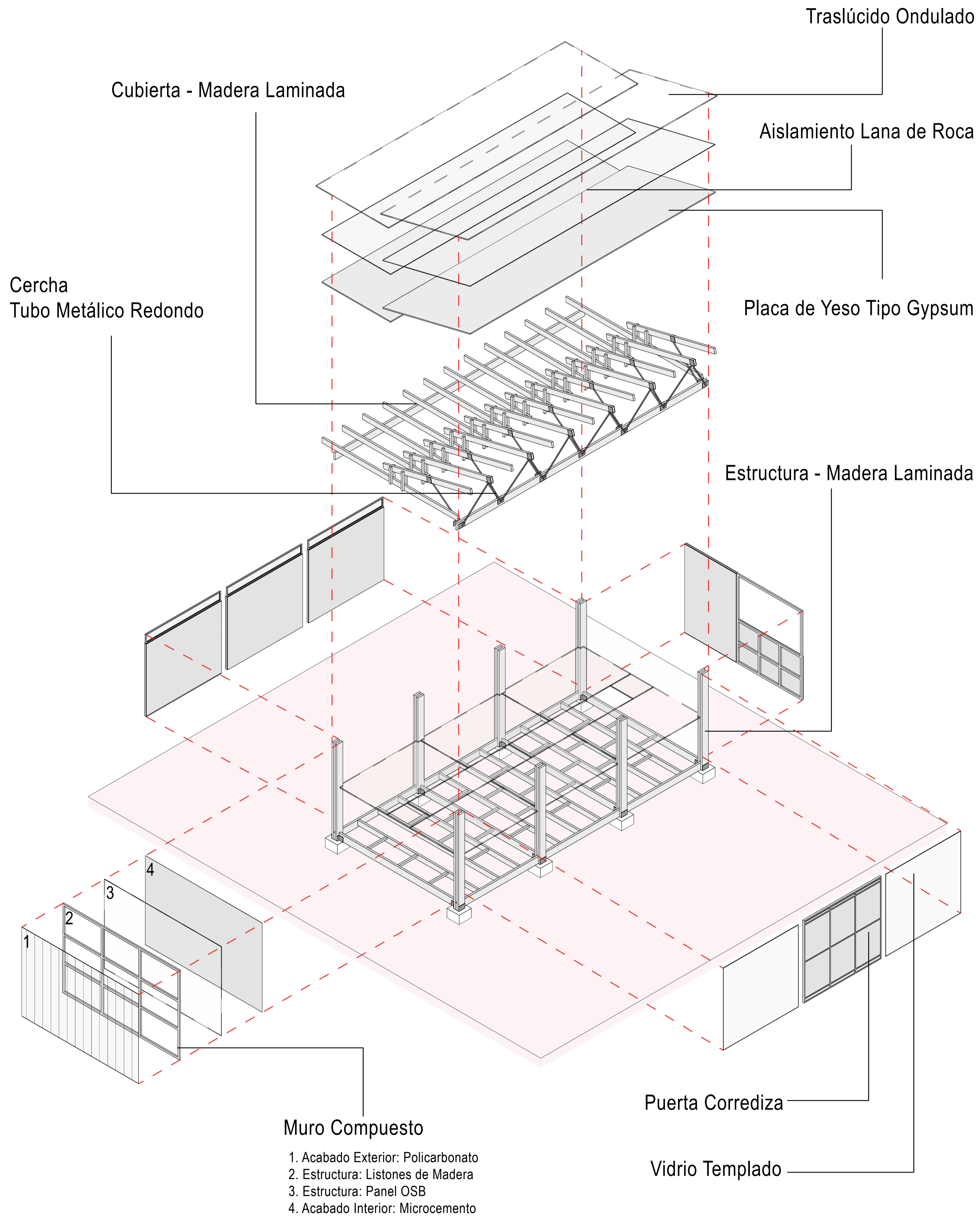
AXONOMETRÍA EXPLOTADA
