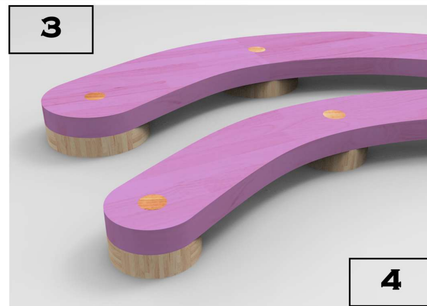
3 4 CADA MÓDULO CURVO DISPONE DE 2 SOPORTES CIRCULARES UNIDOS POR TARUGOS QUE ESTÁN FIJADOS CON COLA DE CARPINTERÍA. EN TOTAL SON 8 SOPORTES DE PINO FINGER JOINT Y 12 TARUGOS DE COIHUE, REVESTIDOS CON BARNIZ PARA MANTENER SU TINTE NATURAL.
