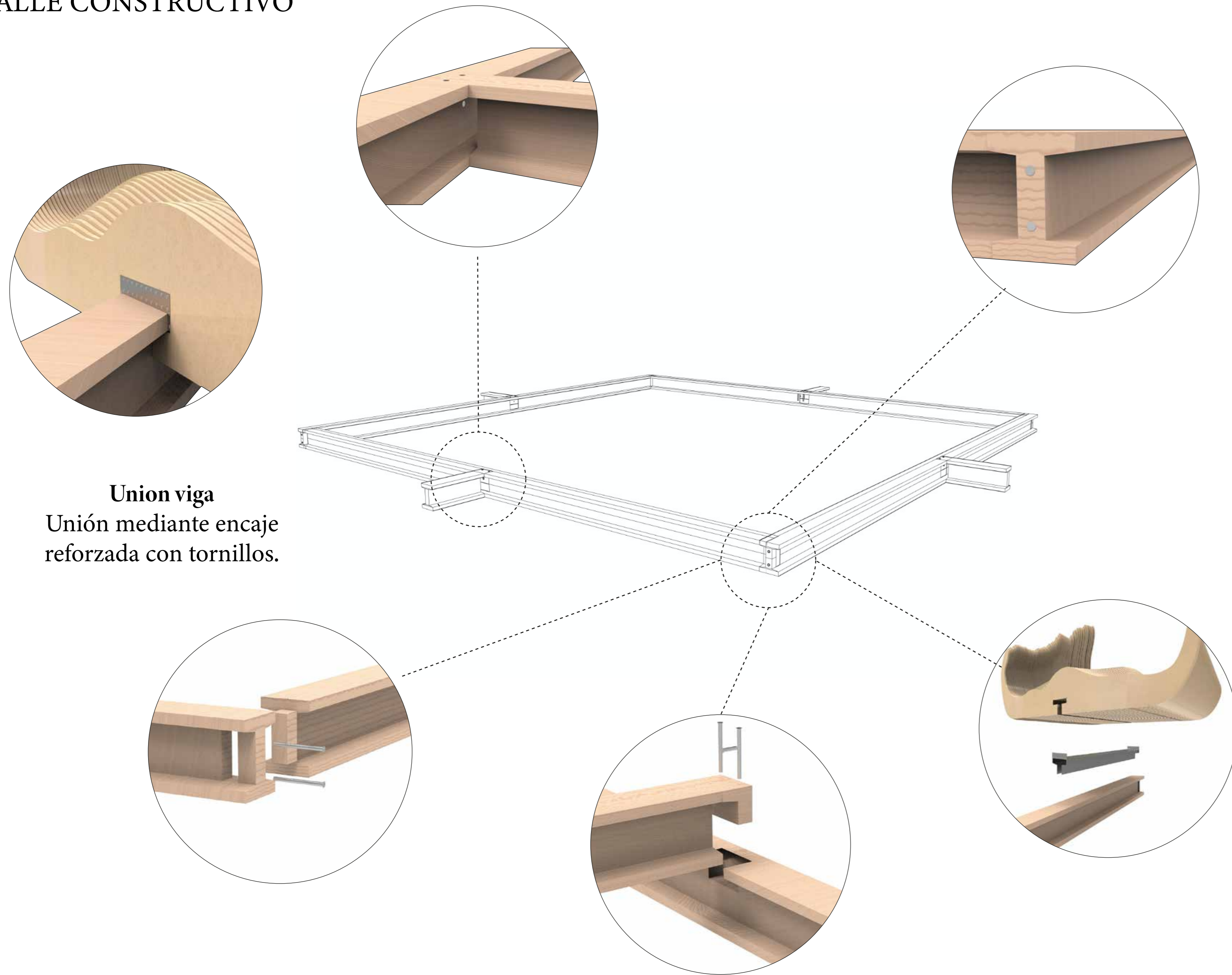
Unión módulo Pieza metálica atornillada a cada extremo del módulo.
