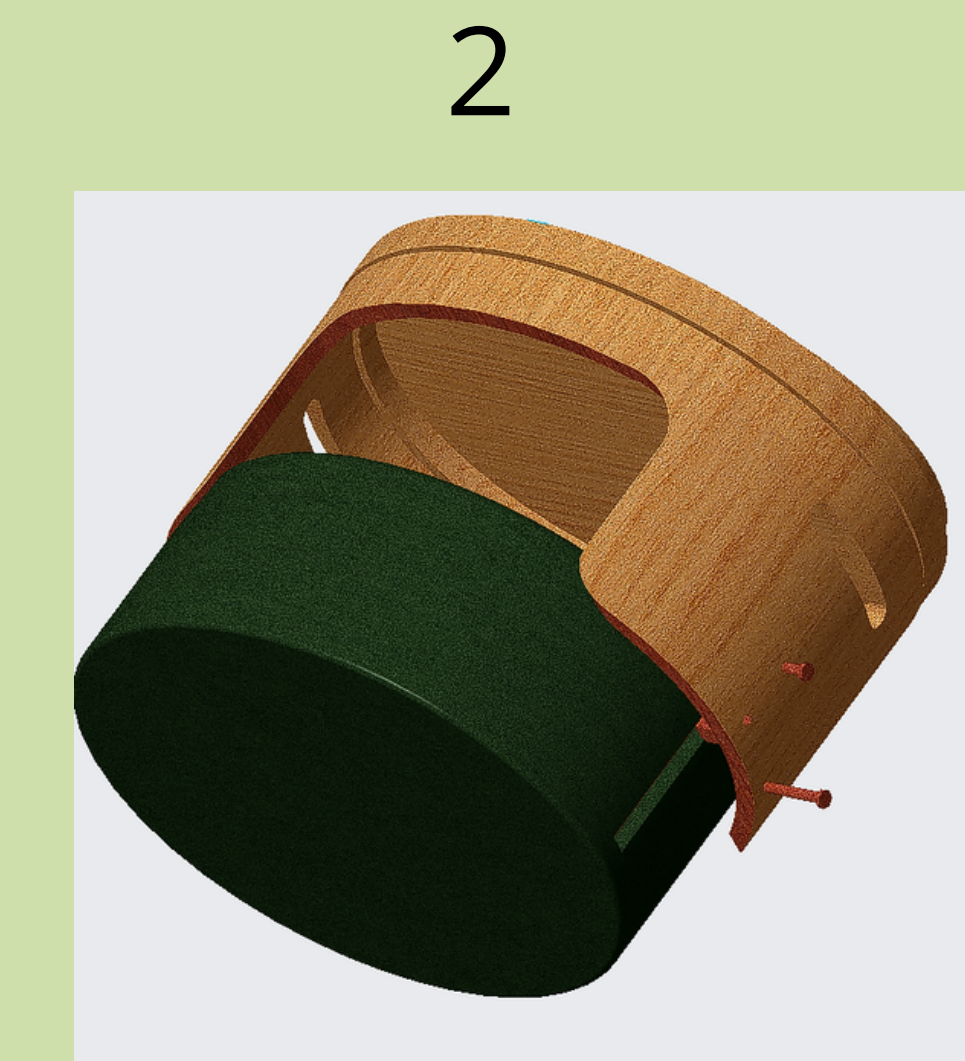
2 Se introduce el felpudo con los encajes laterales interiores de la carcasa
