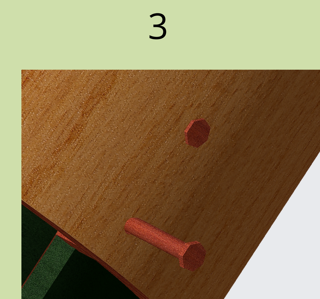
3 Se ponen los tarugos en los orificios laterales exteriores dejando a el felpudo firme dentro de la carcasa.
