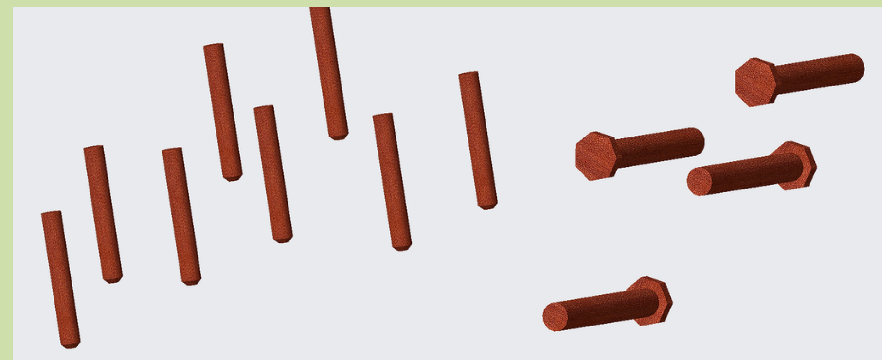
8 pasadores de rauli que mantienen a la tapa y la carcasa alineada y unidas Tarugos de rauli que mantienen sujeto el colchinado a la carcasa con la opción de ser retirados fácilmente.
