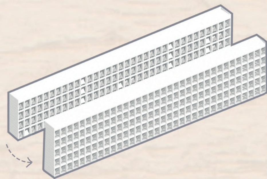
División de dos barras
