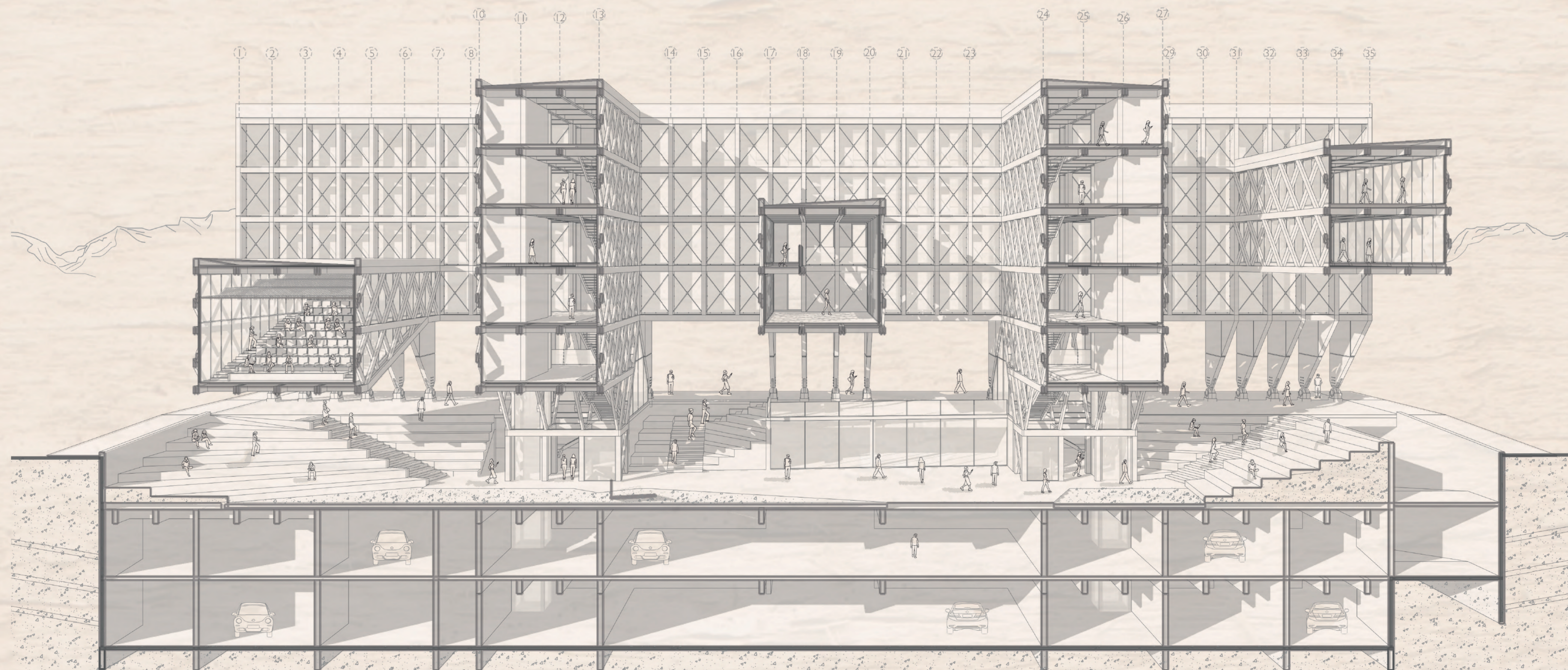
Corte Fugado esc. 1:150
