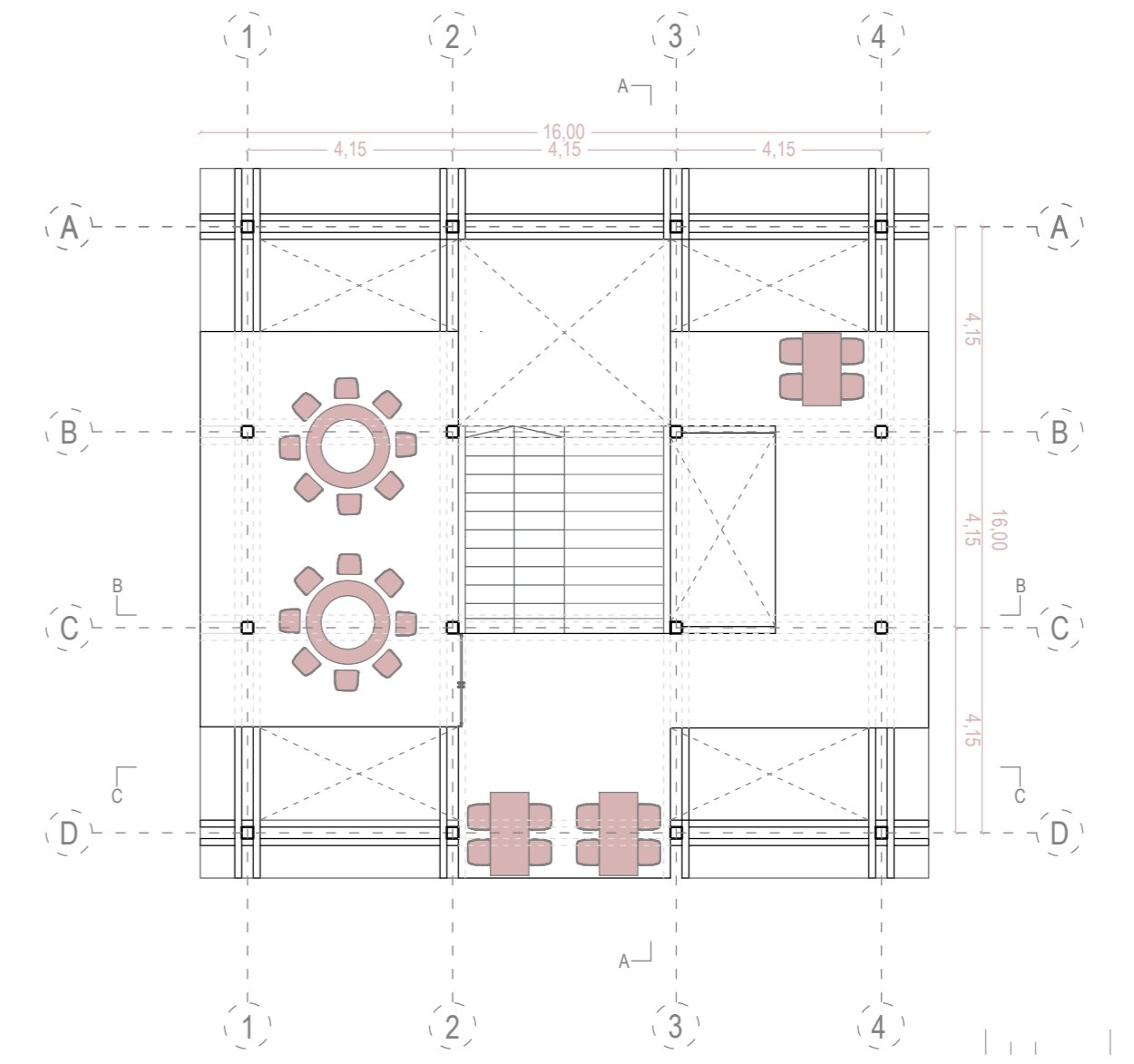
PLANTA 3 ZONAS DE TRABAJOS GRUPALES
