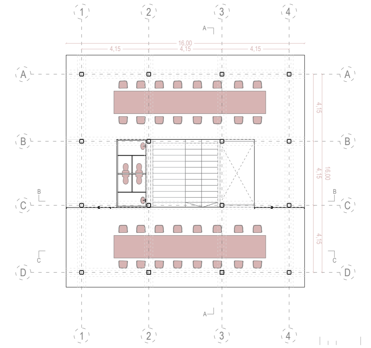
PLANTA 2 TALLER DE ARTESANÍA Y CONFECCIONES
