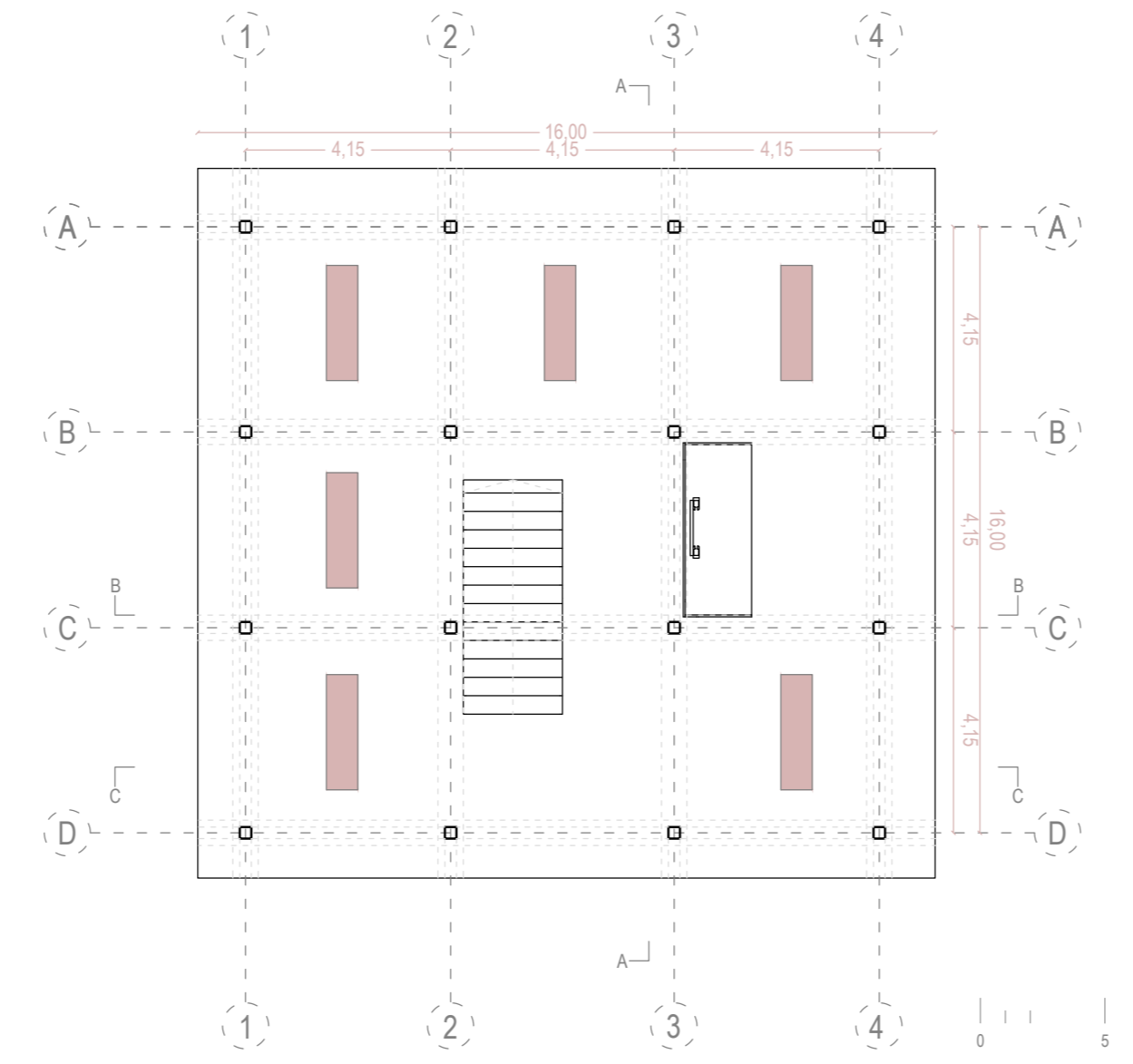
PLANTA 1 ZONA DE EXPOSICIONES
