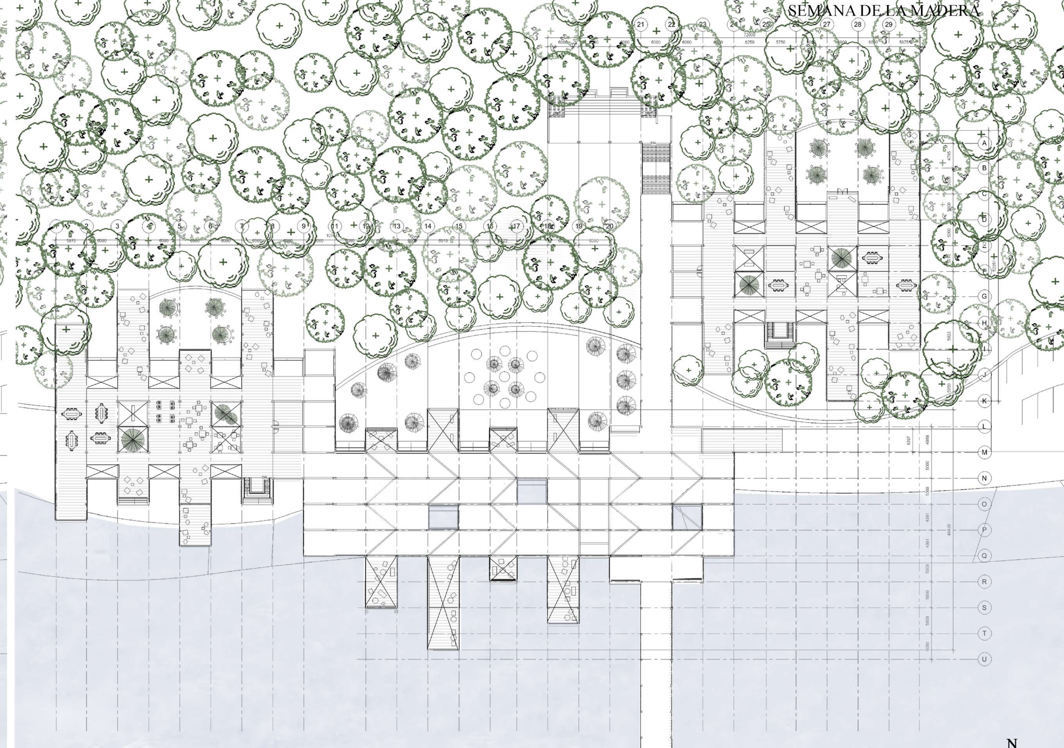
PLANTA 2DO NIVEL 1:400
