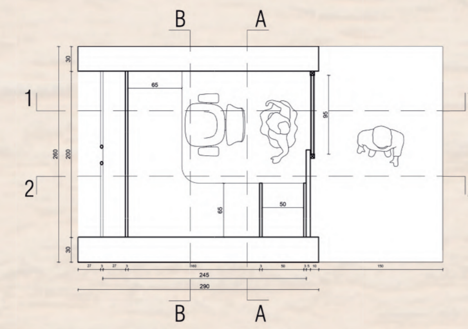
Planta Modulo esc. 1:50
