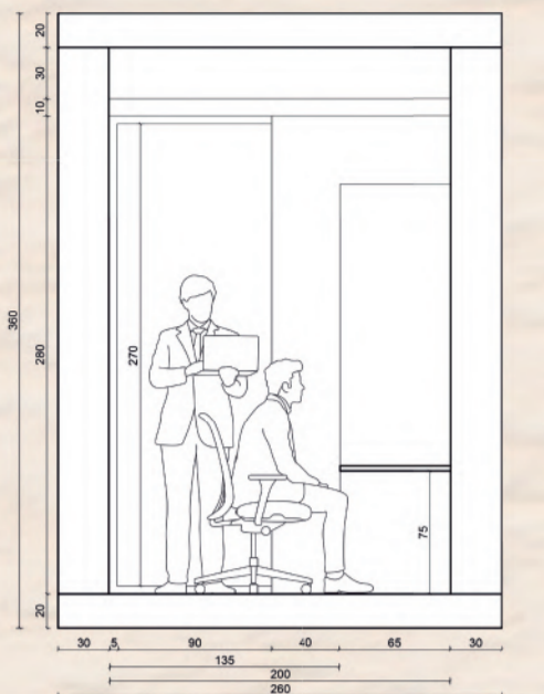
Corte A Modulo esc. 1:50
