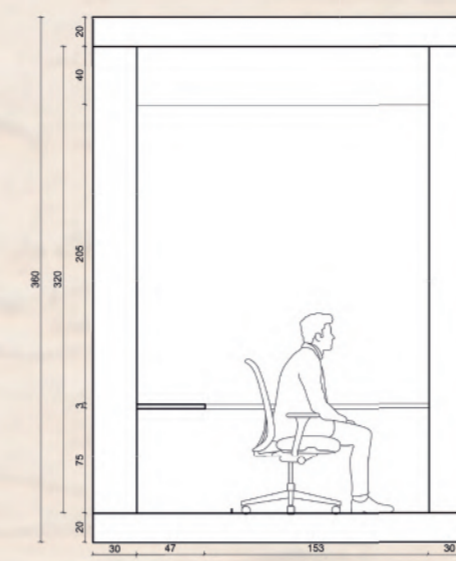
Corte B Modulo esc. 1:50
