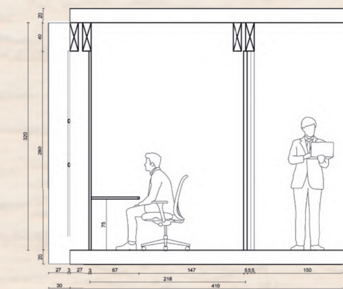
Corte 1 Modulo esc. 1:50
