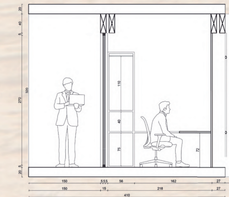
Corte 2 Modulo esc. 1:50
